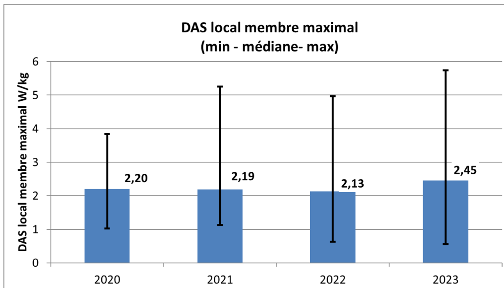
Figure 3 : valeurs médianes, maximales et minimales du DAS membre des téléphones mobiles contrôlés par l'ANFR selon la réglementation en vigueur
