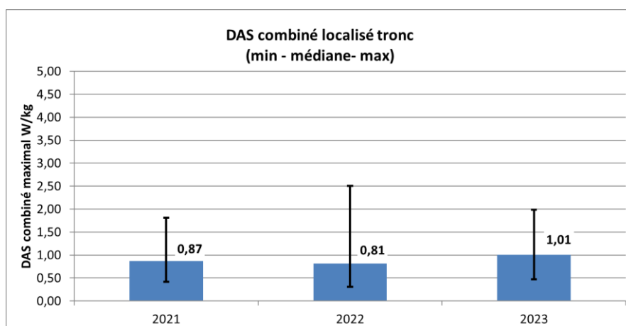
Figure 5 : valeurs médianes, maximales et minimales du DAS combiné tronc des téléphones mobiles contrôlés par l'ANFR selon la réglementation en vigueur
