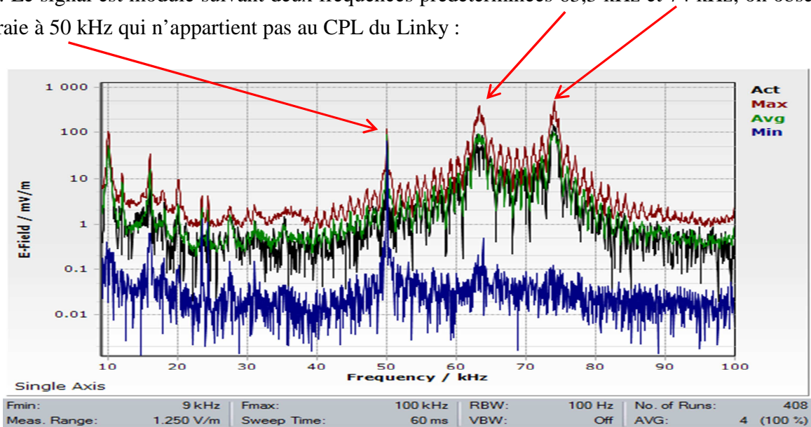
L'analyse spectrale du champ électrique à 20 cm du compteur
