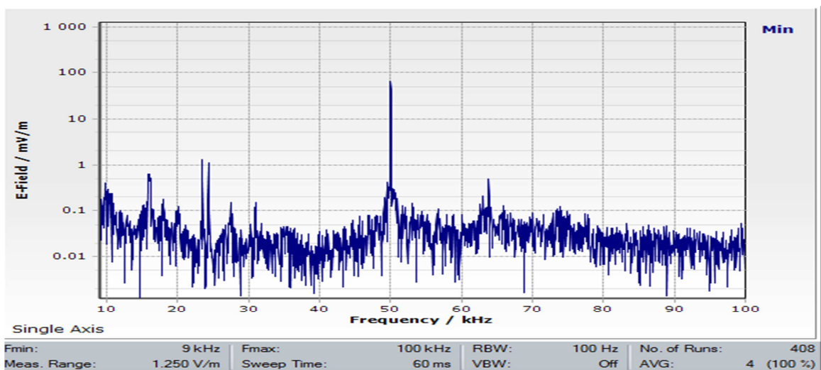
Spectre entre 2 trames LINKY
