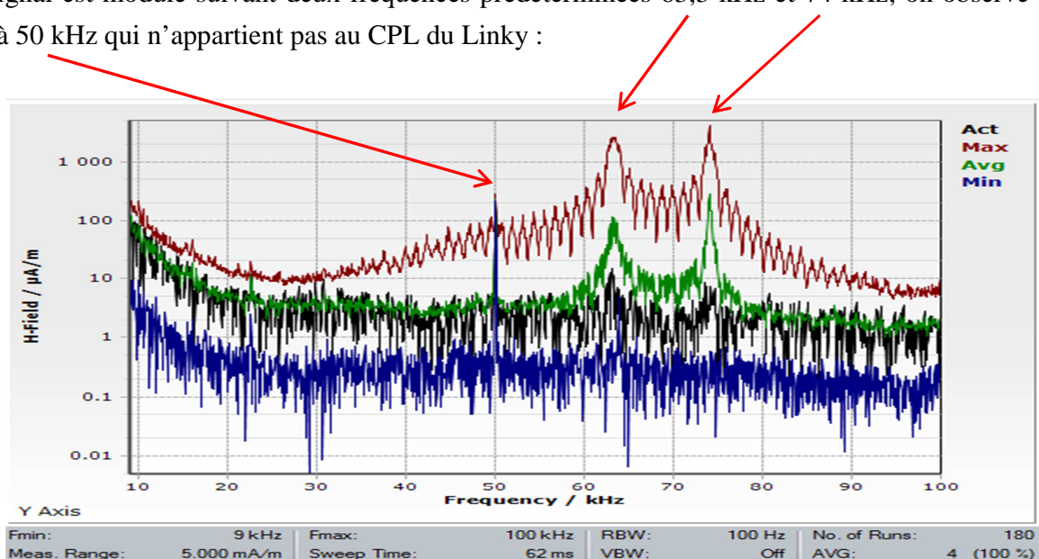
L'analyse spectrale du champ magnétique à 20 cm du compteur
