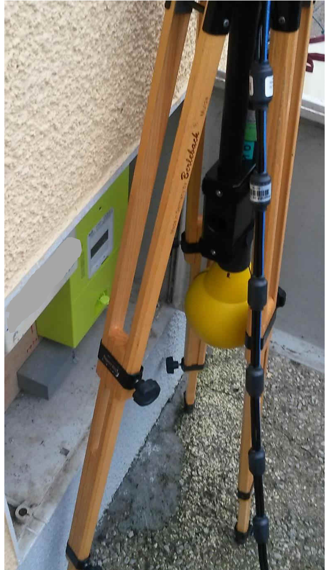
Mesure avec l'antenne électrique puis magnétique devant le compteur
