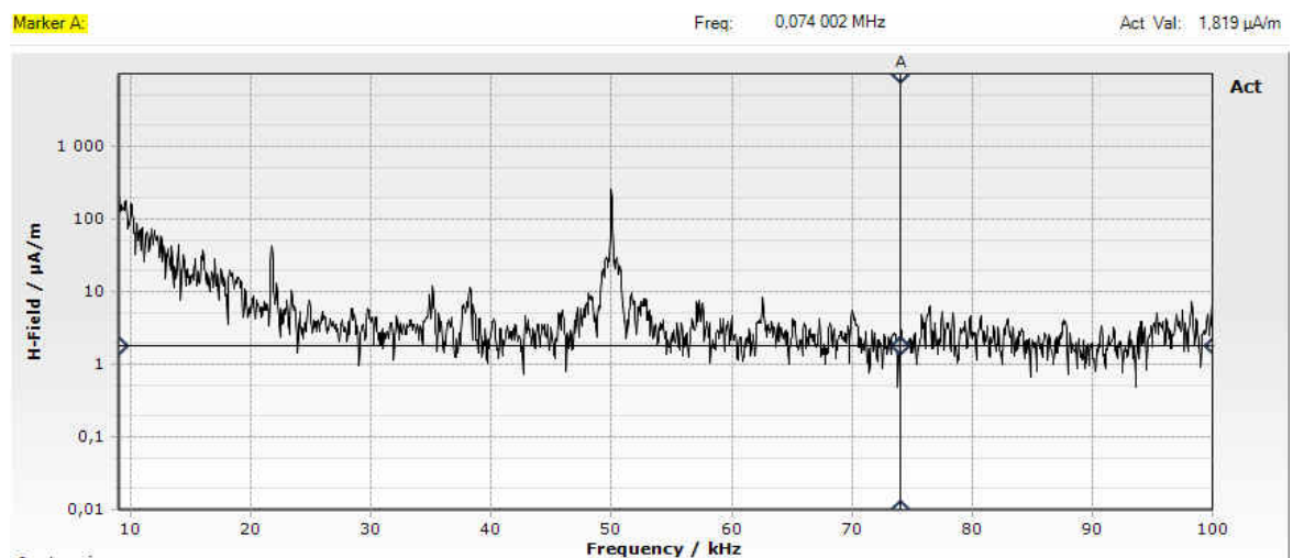
Le spectre entre deux salves Linky
