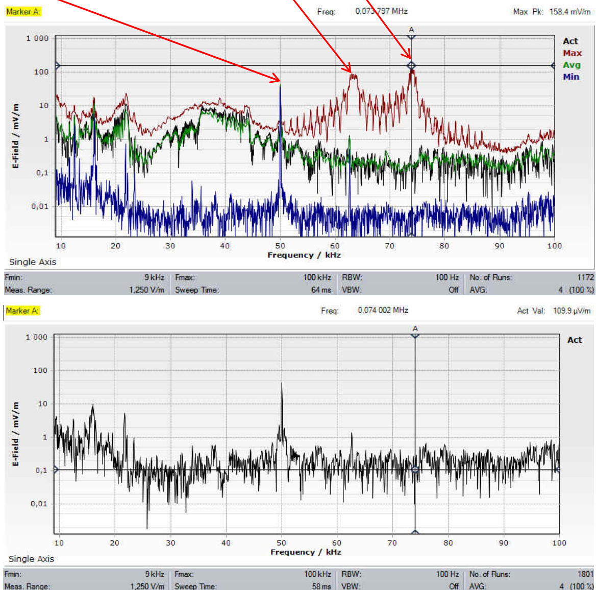
Le spectre entre deux salves Linky
