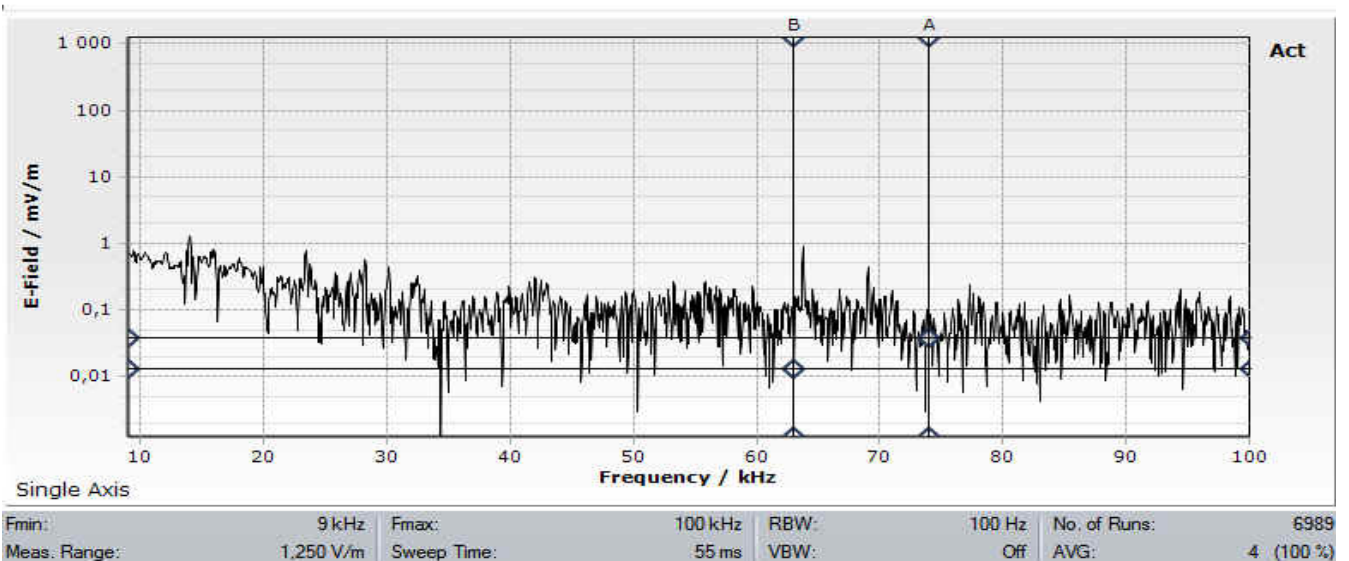
Le spectre entre deux salves Linky
