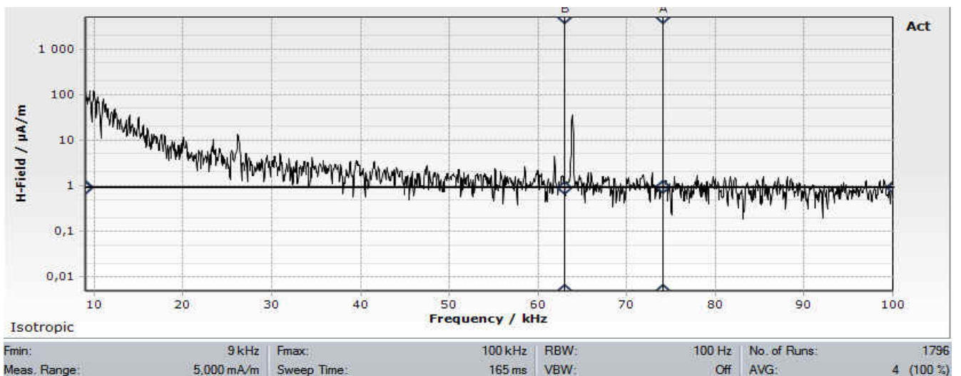
Le spectre entre deux salves Linky
