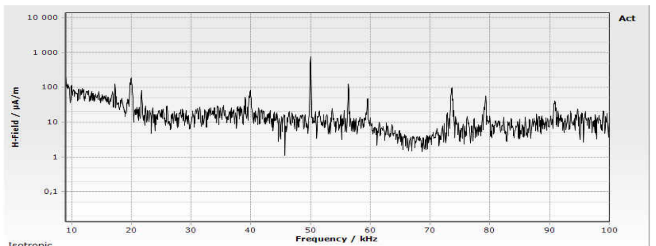
Le spectre entre deux salves Linky
