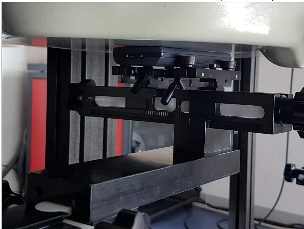
Photo 8: Position d'essai face avant contre le membre (distance 0 mm)
