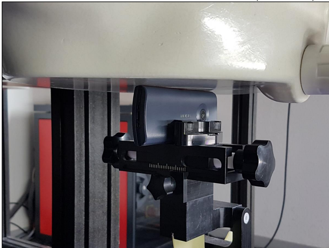
Photo 11: Position d'essai face du côté droite contre le membre (distance 0 mm)
