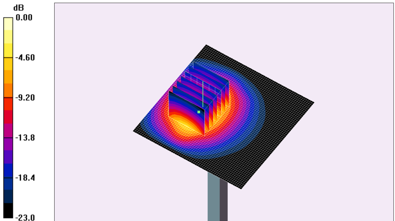
Fig. 7 : Résultat de la vérification à 2450MHz
