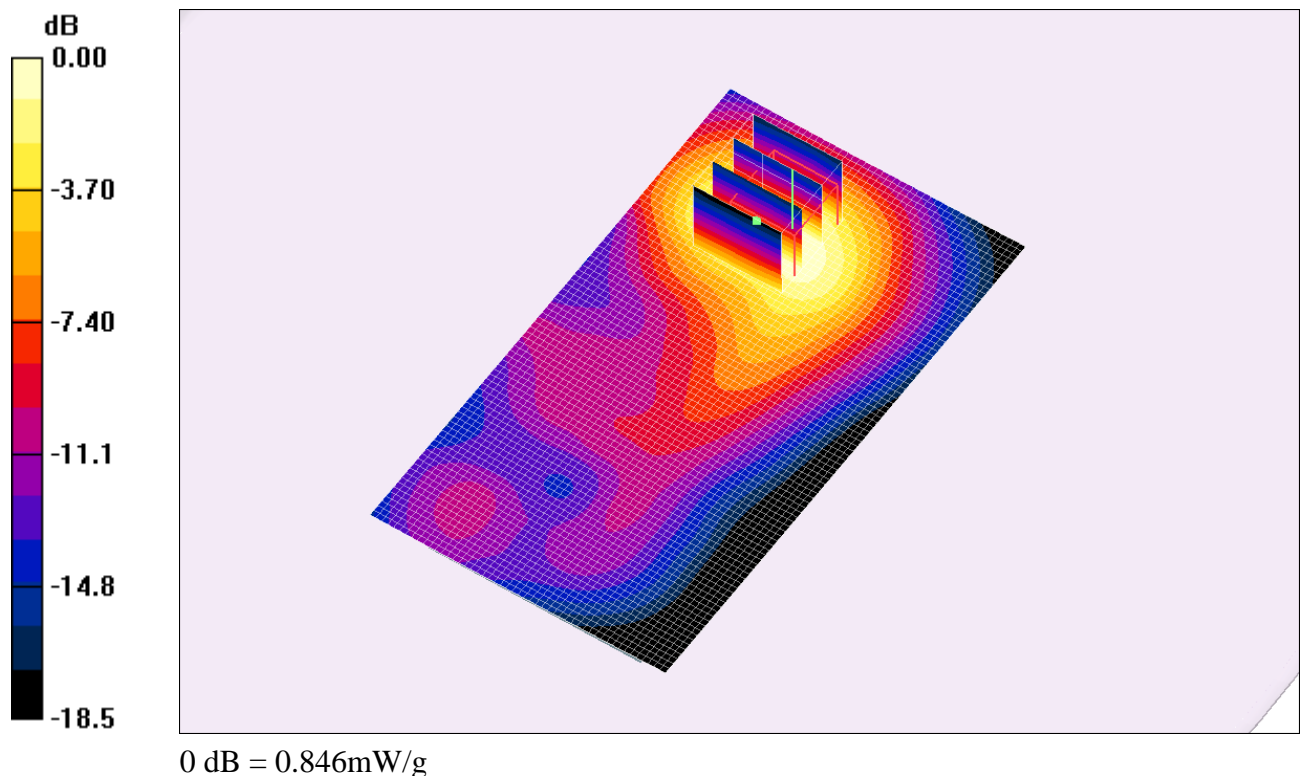
Fig. 14 : Distribution du DAS en LTE 2600: canal 20775 (2502.5 MHz) face arrière à 1.5cm du fantôme
