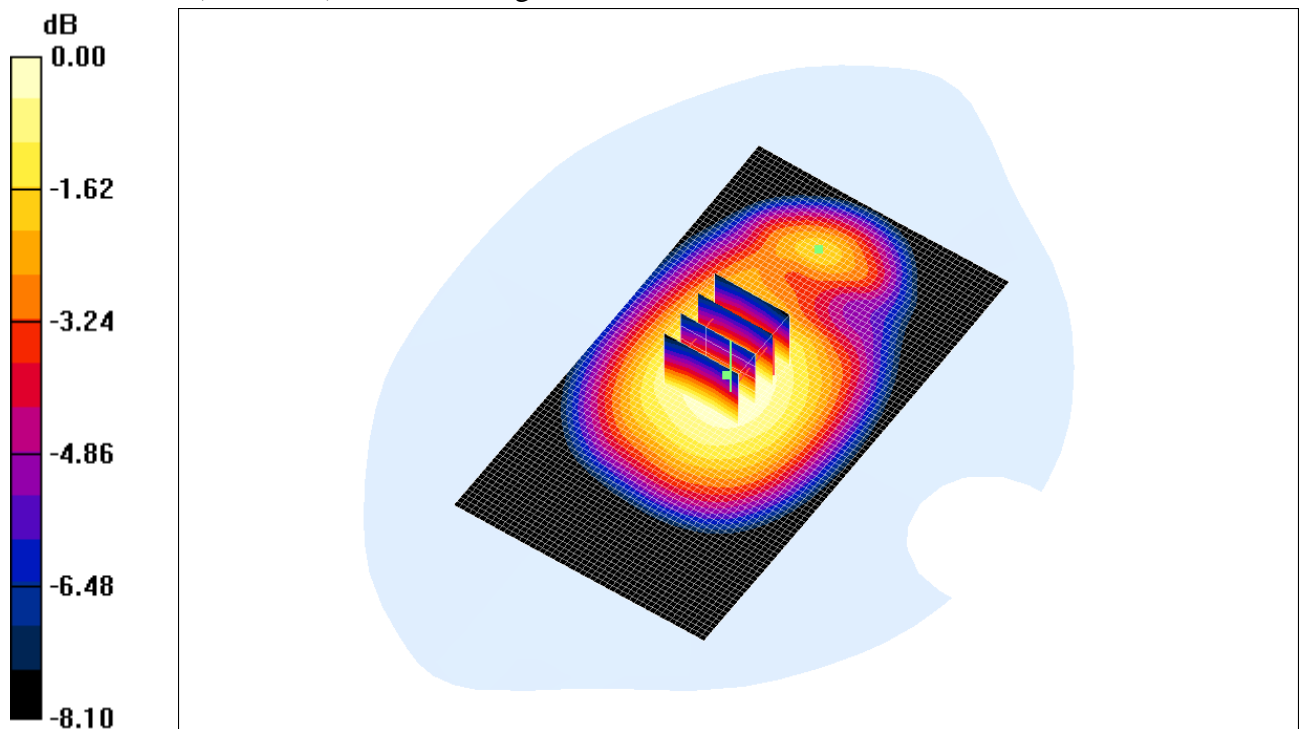
Fig. 8 : Distribution du DAS en GSM-GPRS 900: canal 038 (897.6 MHz) face arrière à 1.5cm du fantôme
