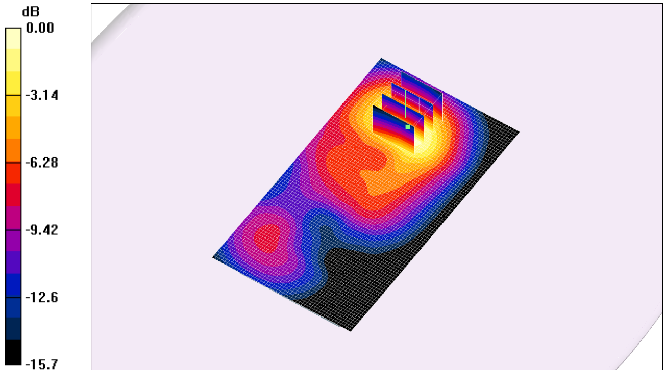
Fig. 11 : Distribution du DAS en WCDMA 2100: canal 9888 (1977.6 MHz) face arrière à 1.5cm du fantôme
