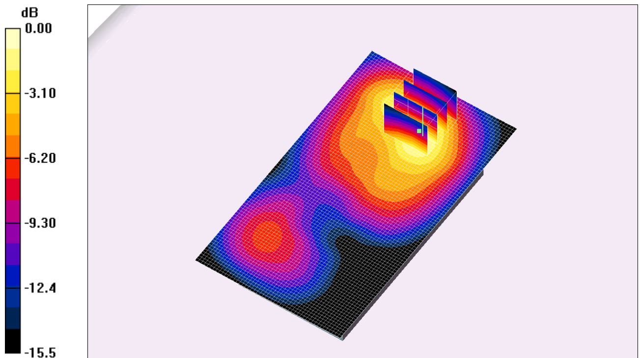
Fig. 13 : Distribution du DAS en LTE 1800: canal 19925 (1782.5 MHz) face arrière à 1.5cm du fantôme
