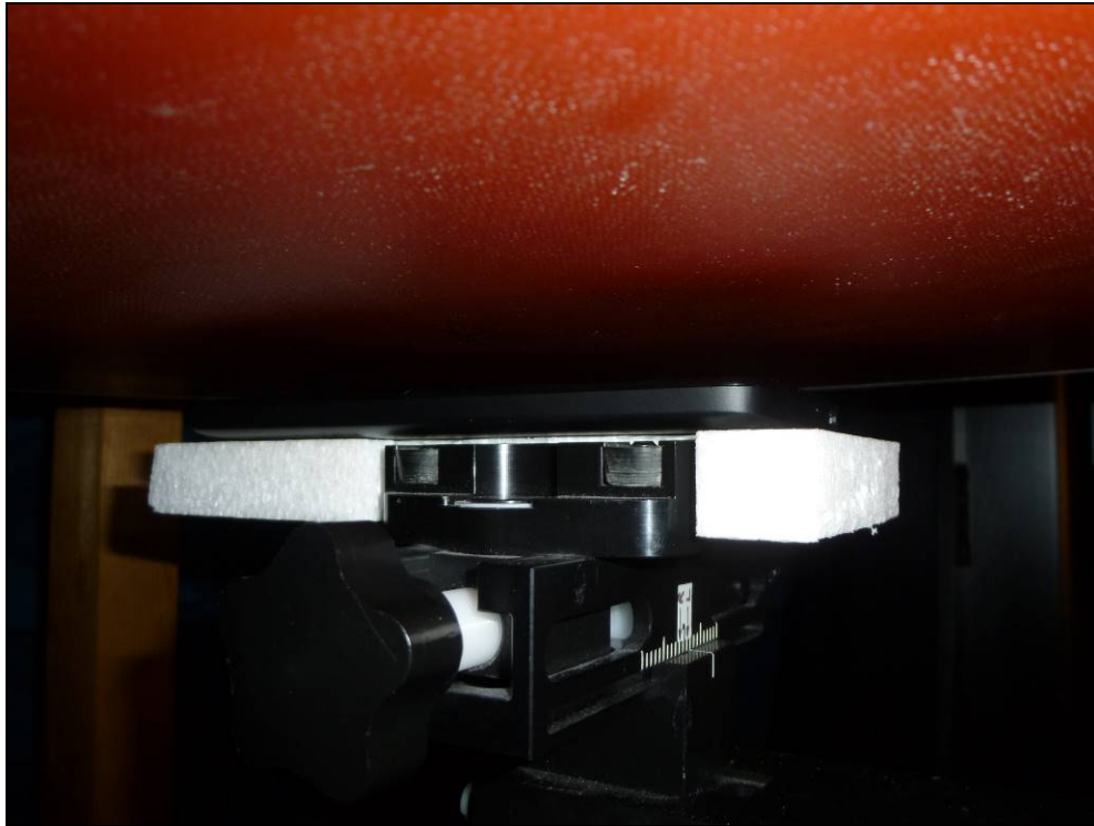
Fig. 17 : Face avant à 1.5cm du fantôme ELI4
