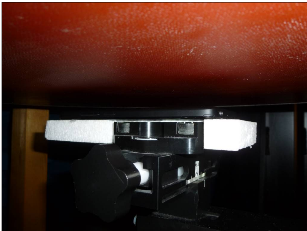
Fig. 18 : Face arrière à 1.5cm du fantôme ELI4
