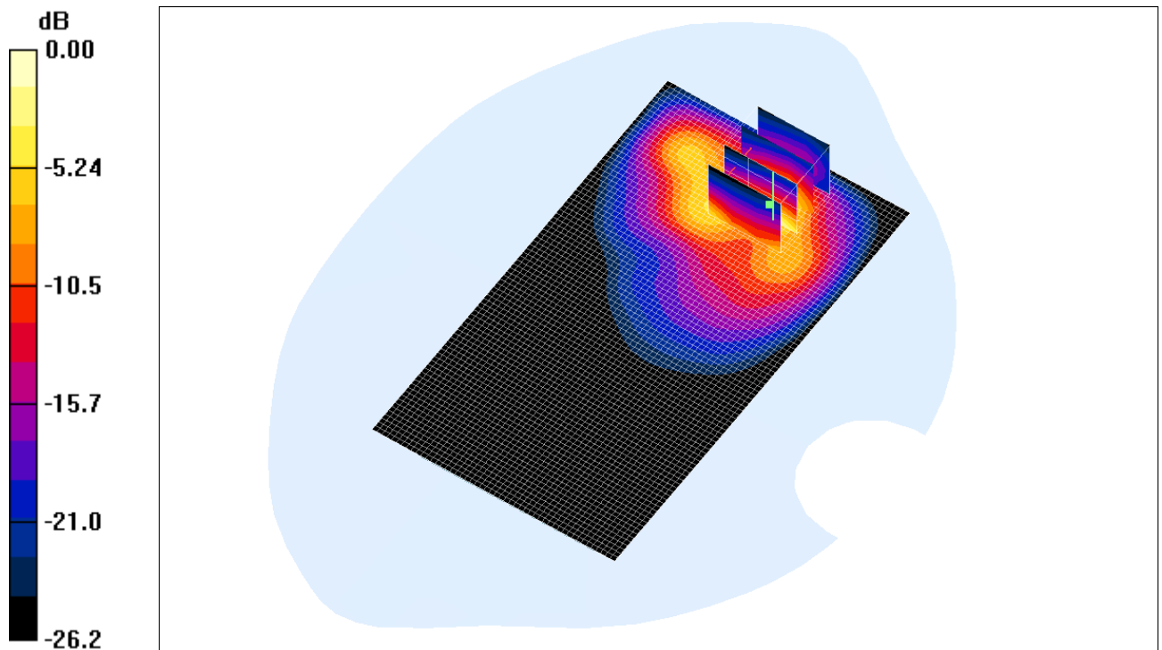
Fig. 14: Distribution du DAS en LTE 2600: canal 21425 (2567.5 MHz) face arrière à 0cm du fantôme
