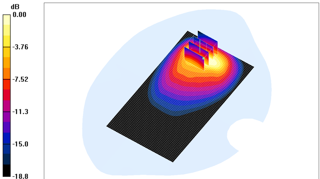
Fig. 8: Distribution du DAS en GSM-GPRS 900: canal 038 (897.6 MHz) face arrière à 0cm du fantôme
