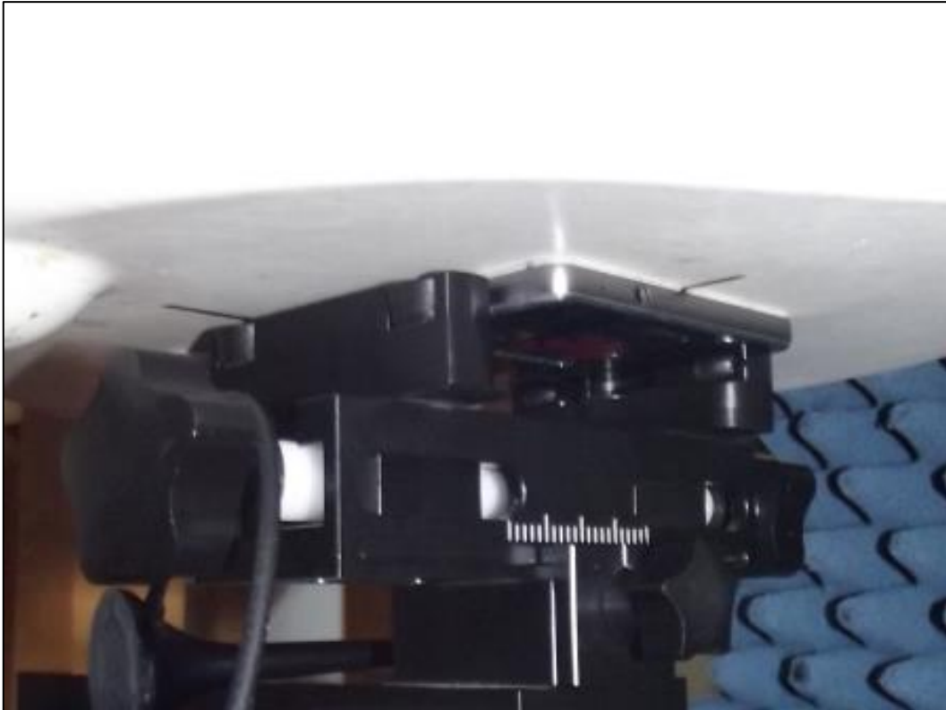
Photo 7: Position d'essai face arrière contre le corps (distance 0 mm)
