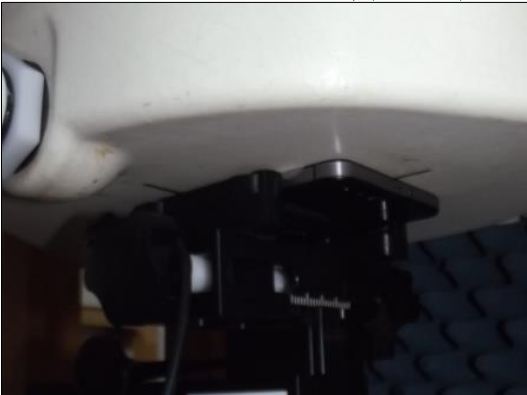
Photo 6: Position d'essai face avant contre le corps (distance 0 mm)
