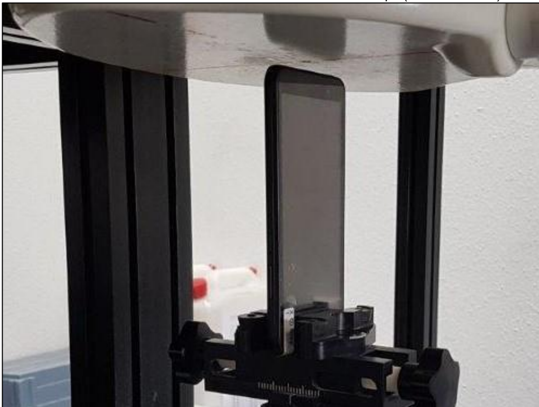
Photo 14: Position d'essai face du dessous contre le corps (distance 5 mm)
