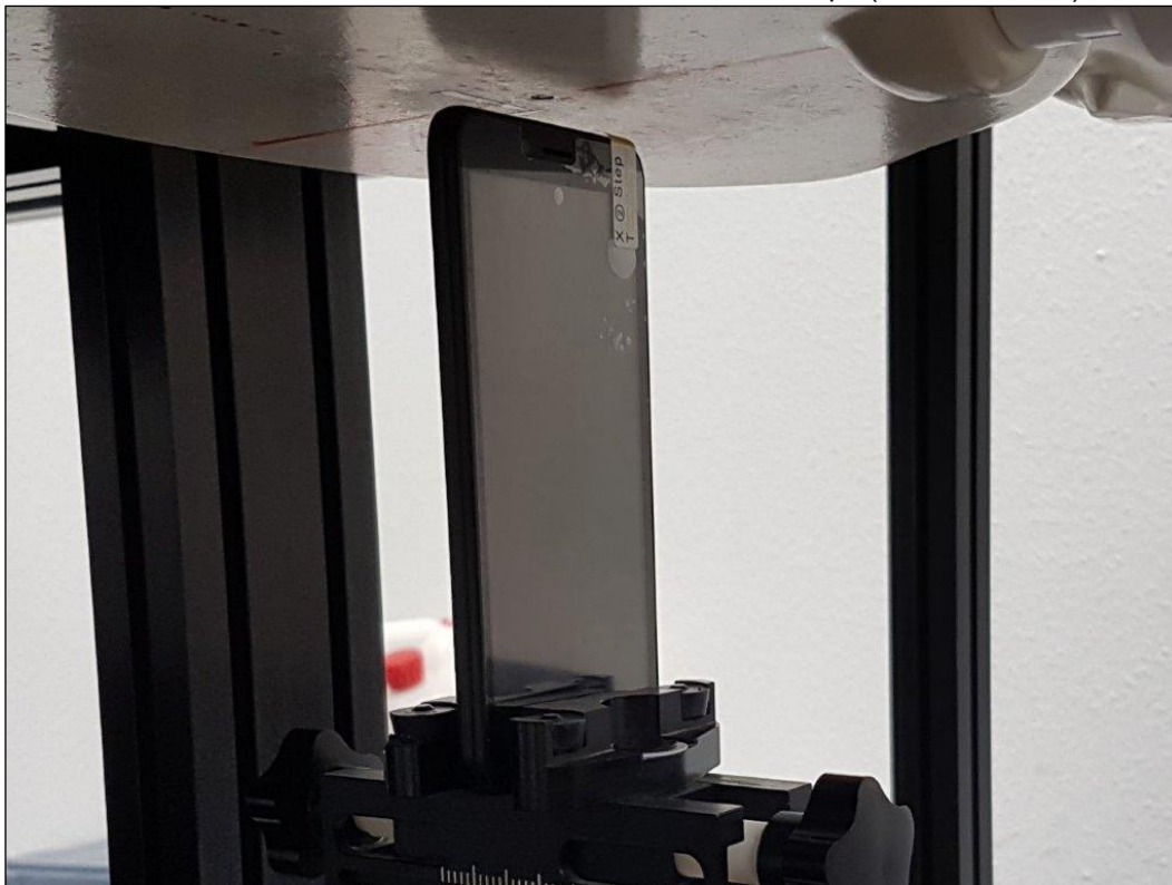
Photo 13: Position d'essai face du dessus contre le corps (distance 5 mm)
