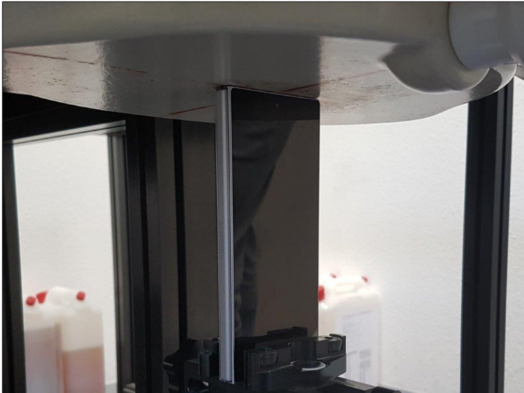
Photo 17: Position d'essai face du dessus pilé contre le membre (distance 0 mm)
