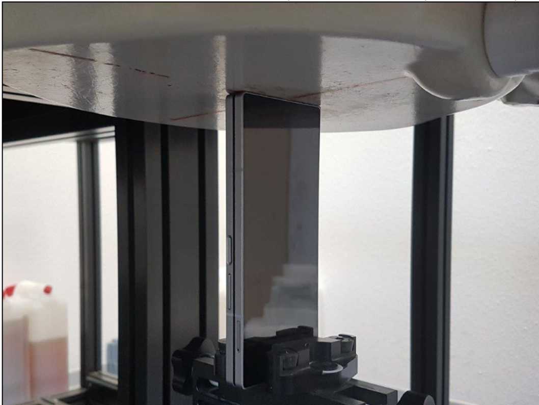
Photo 18: Position d'essai face du dessous pilé contre le membre (distance 0 mm)
