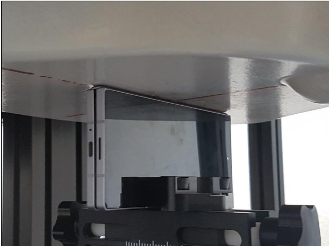
Photo 15: Position d'essai face du côté gauche pilé contre le membre (distance 0 mm)
