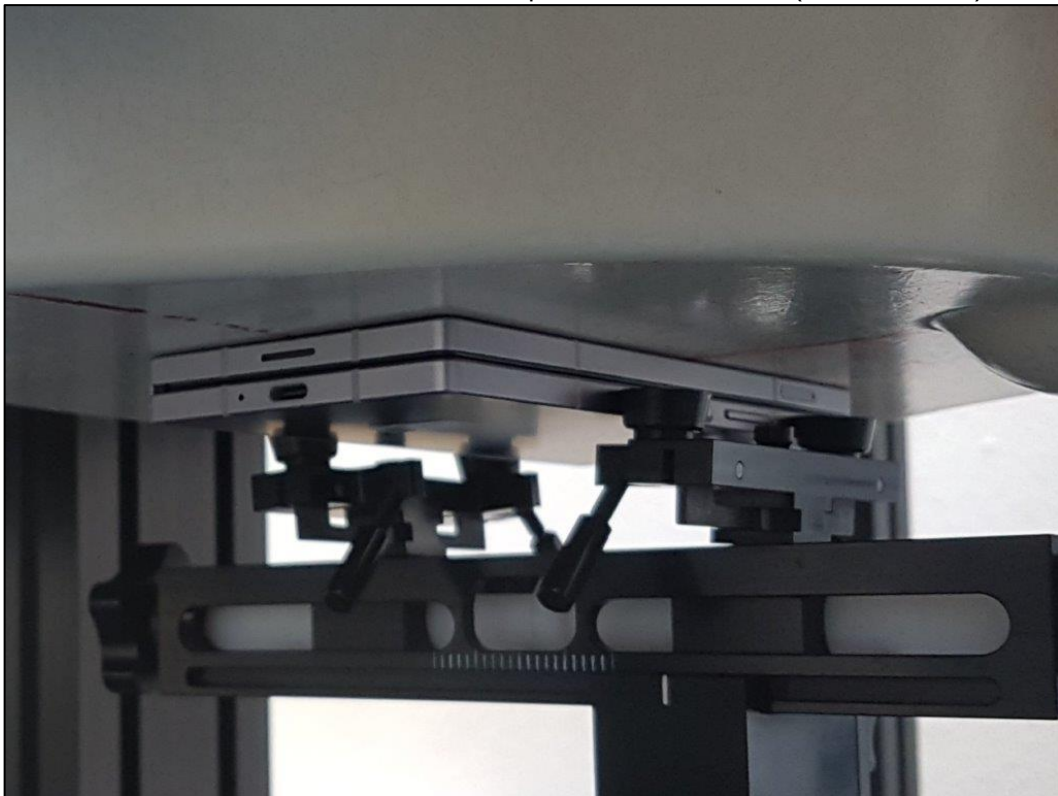
Photo 13: Position d'essai face avant pilé contre le membre (distance 0 mm)
