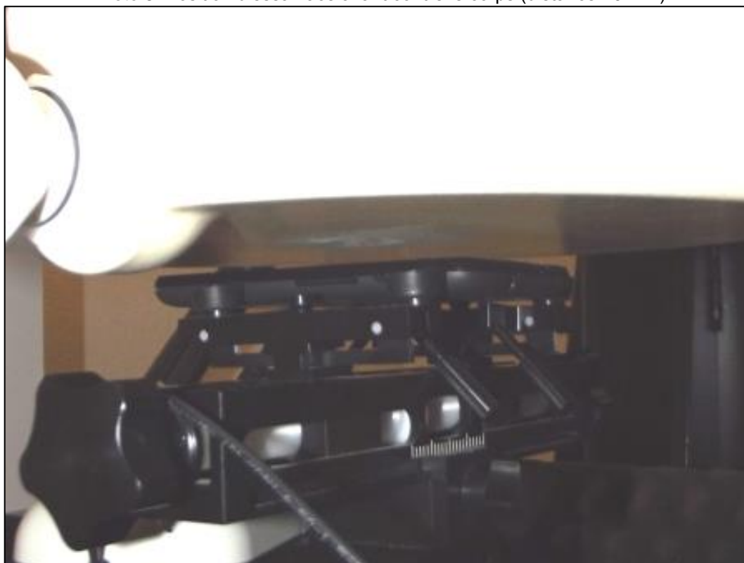
Photo 8: Position d'essai face avant contre le corps (distance 10 mm)
