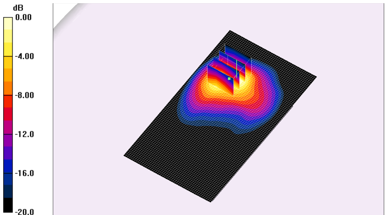
Fig. 18: Distribution du DAS en LTE 1800: canal 19575 (1747.5 MHz) face arrière à 0cm du fantôme
