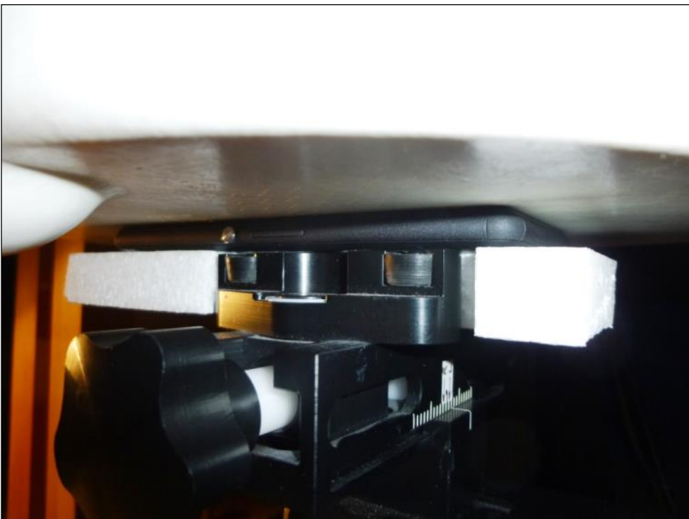
Fig. 24: Face arrière à 0cm des fantômes ELI4 et SAM
