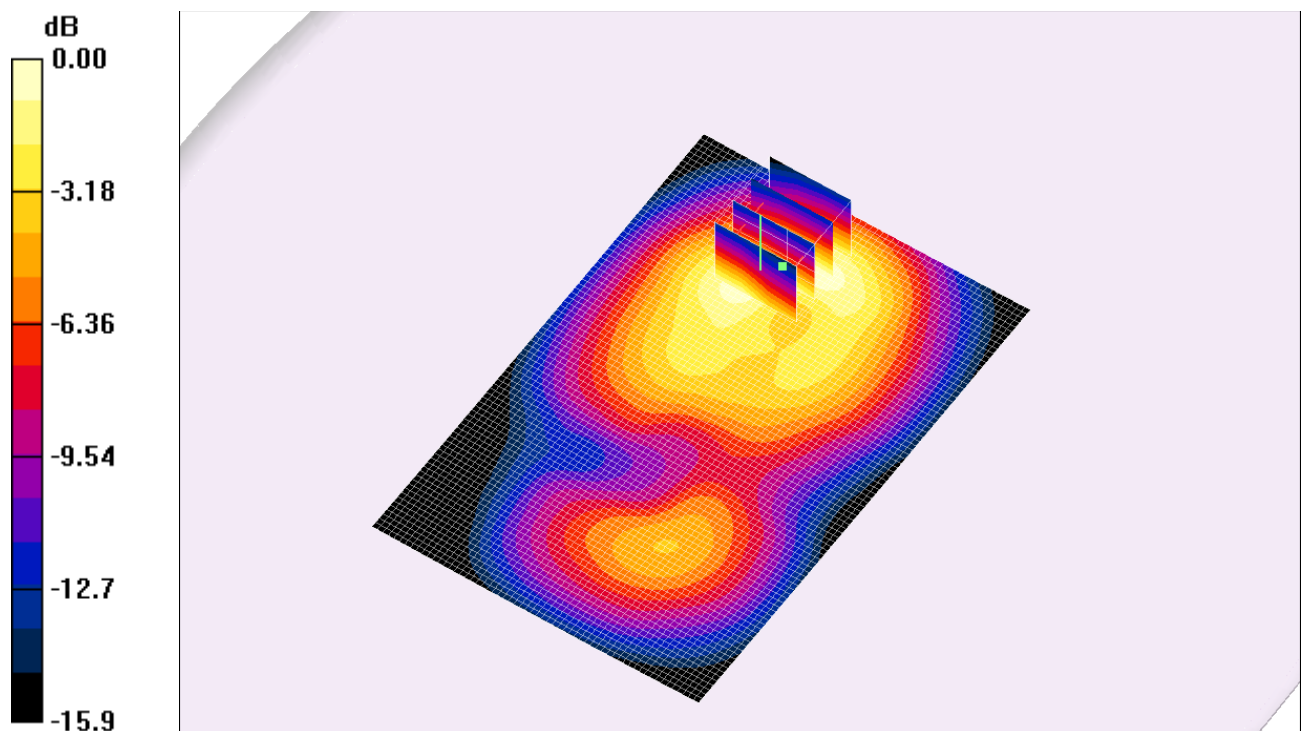
Fig. 15: Distribution du DAS en WCDMA 2100: canal 9750 (1950.0 MHz) face arrière à 1.5cm du fantôme
