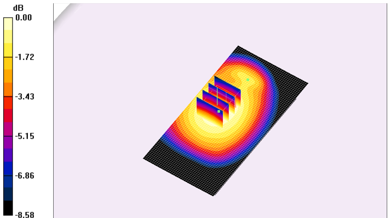
Fig. 13: Distribution du DAS en WCDMA 900: canal 2788 (897.6 MHz) face arrière à 1.5cm du fantôme
