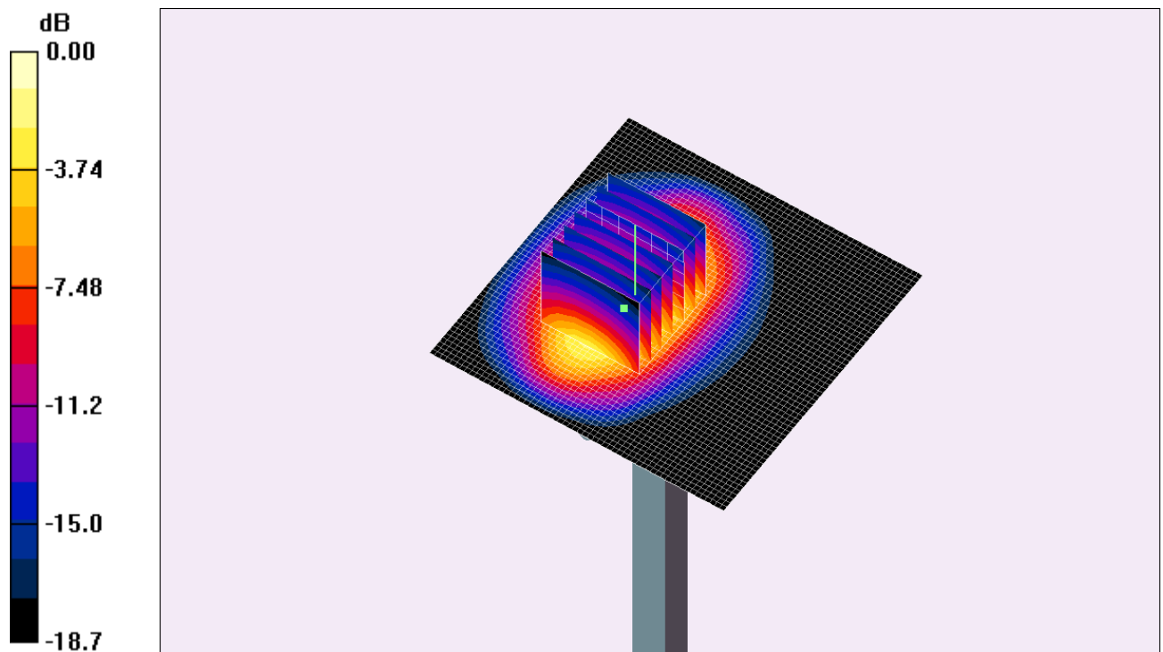
Fig. 6: Résultat de la validation à 1950MHz
