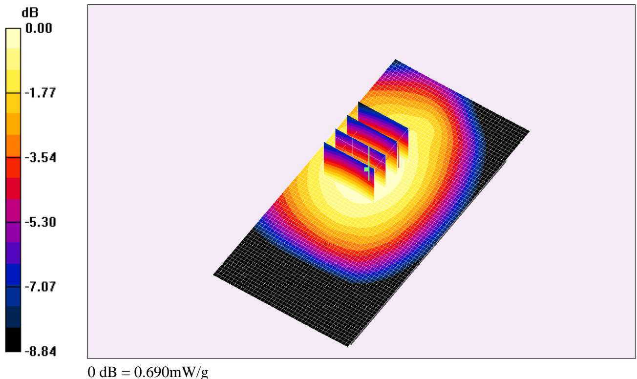
Fig. 9: Distribution du DAS en GSM-GPRS 900: canal 038 (897.6 MHz) face arrière à 1.5cm du fantôme
