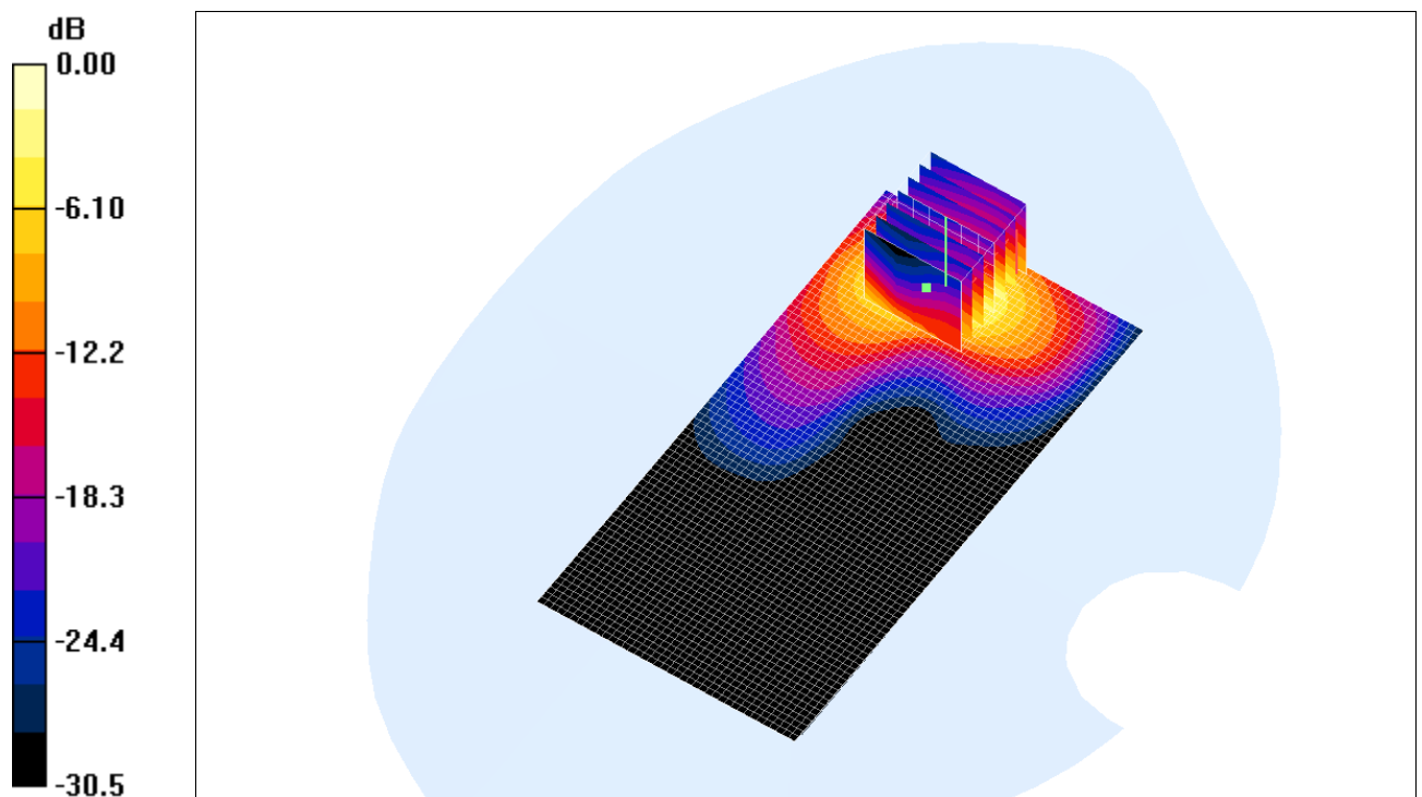
Fig. 21: Distribution du DAS en LTE 2600: canal 21100 (2535.0 MHz) face arrière à 0cm du fantôme Mesure avec balayage zoom normatif
