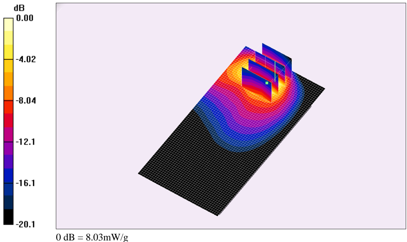
Fig. 8: Distribution du DAS en GSM-GPRS 900: canal 038 (897.6 MHz) face arrière à 0cm du fantôme
