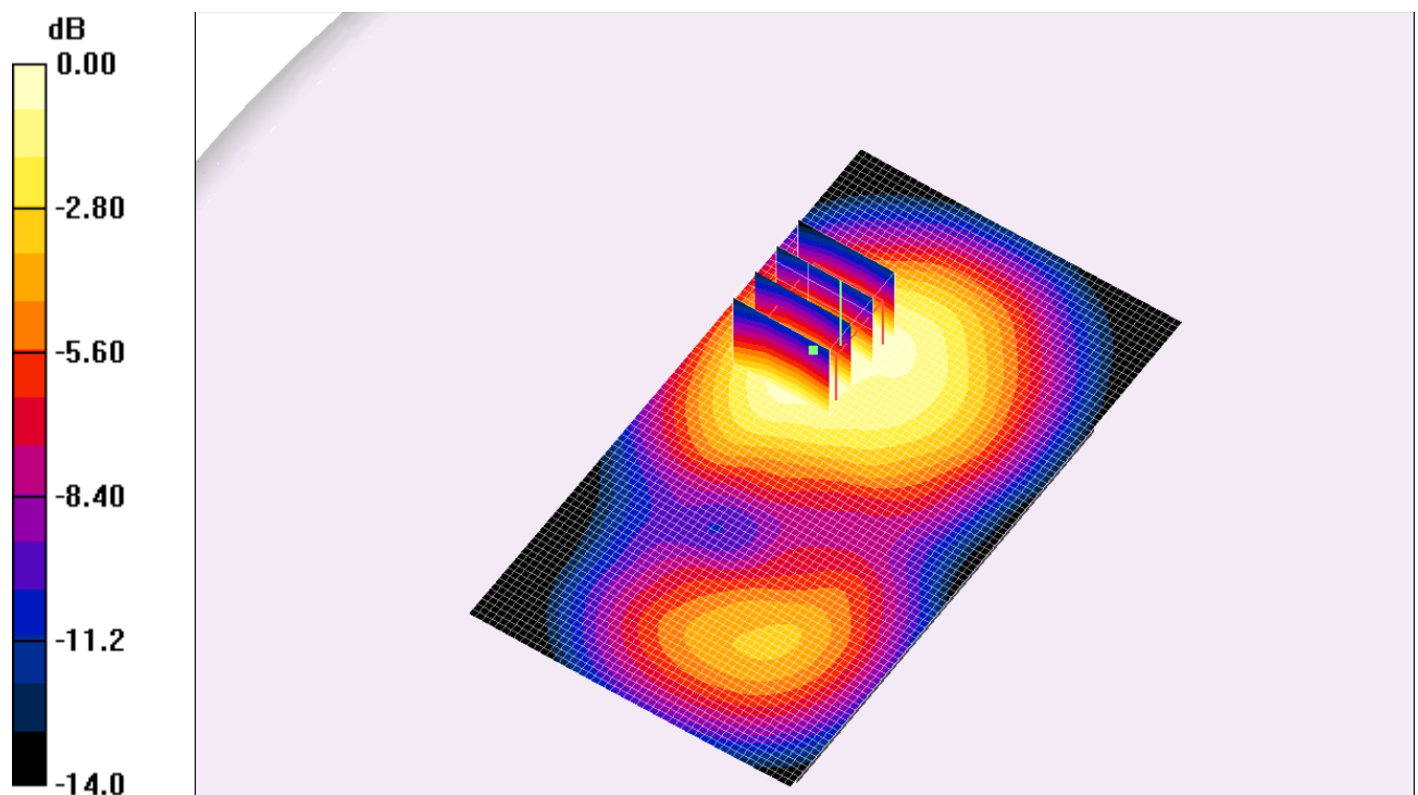
Fig. 19: Distribution du DAS en LTE 1800: canal 19575 (1747.5 MHz) face arrière à 1.5cm du fantôme
