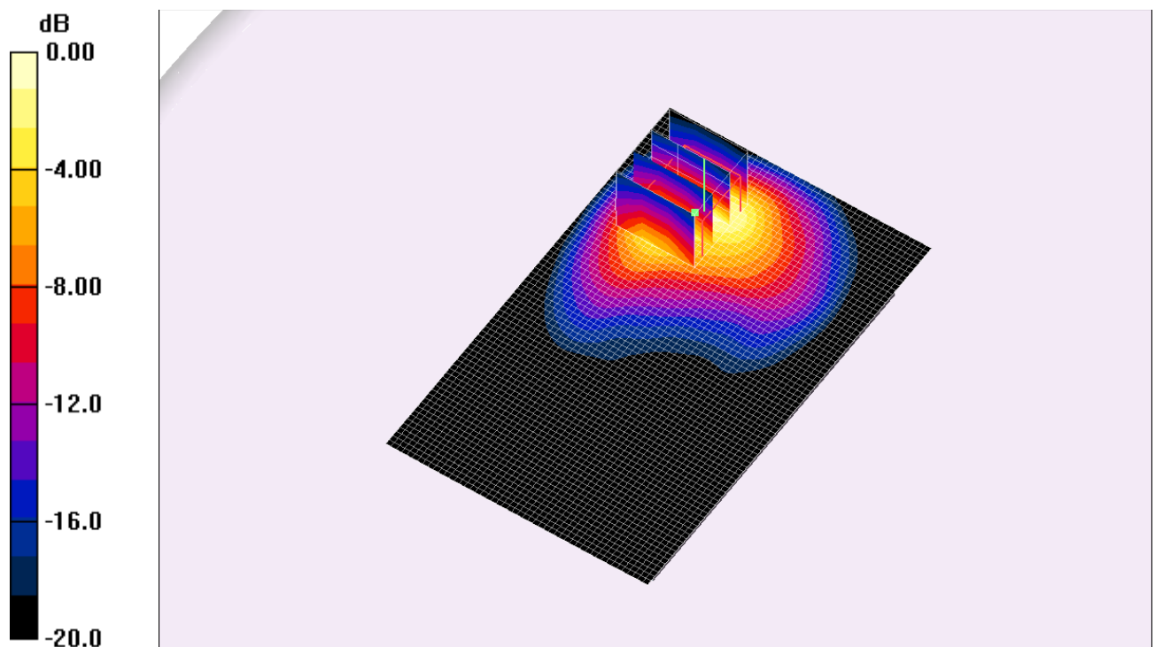
Fig. 10: Distribution du DAS en GSM-GPRS 1800: canal 699 (1747.6 MHz) face arrière à 0cm du fantôme
