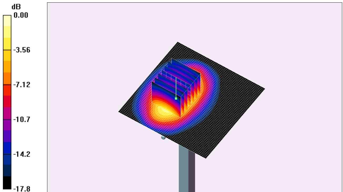
Fig. 5: Résultat de la validation à 1800MHz
