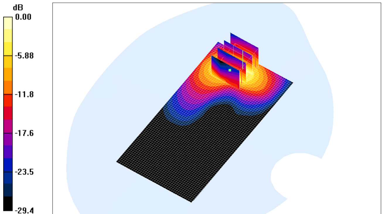
Fig. 20: Distribution du DAS en LTE 2600: canal 21100 (2535.0 MHz) face arrière à 0cm du fantôme
