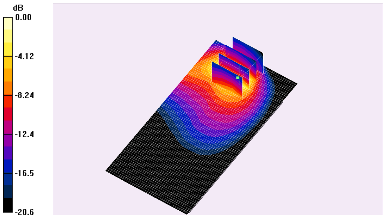
Fig. 12: Distribution du DAS en WCDMA 900: canal 2788 (897.6 MHz) face arrière à 0cm du fantôme
