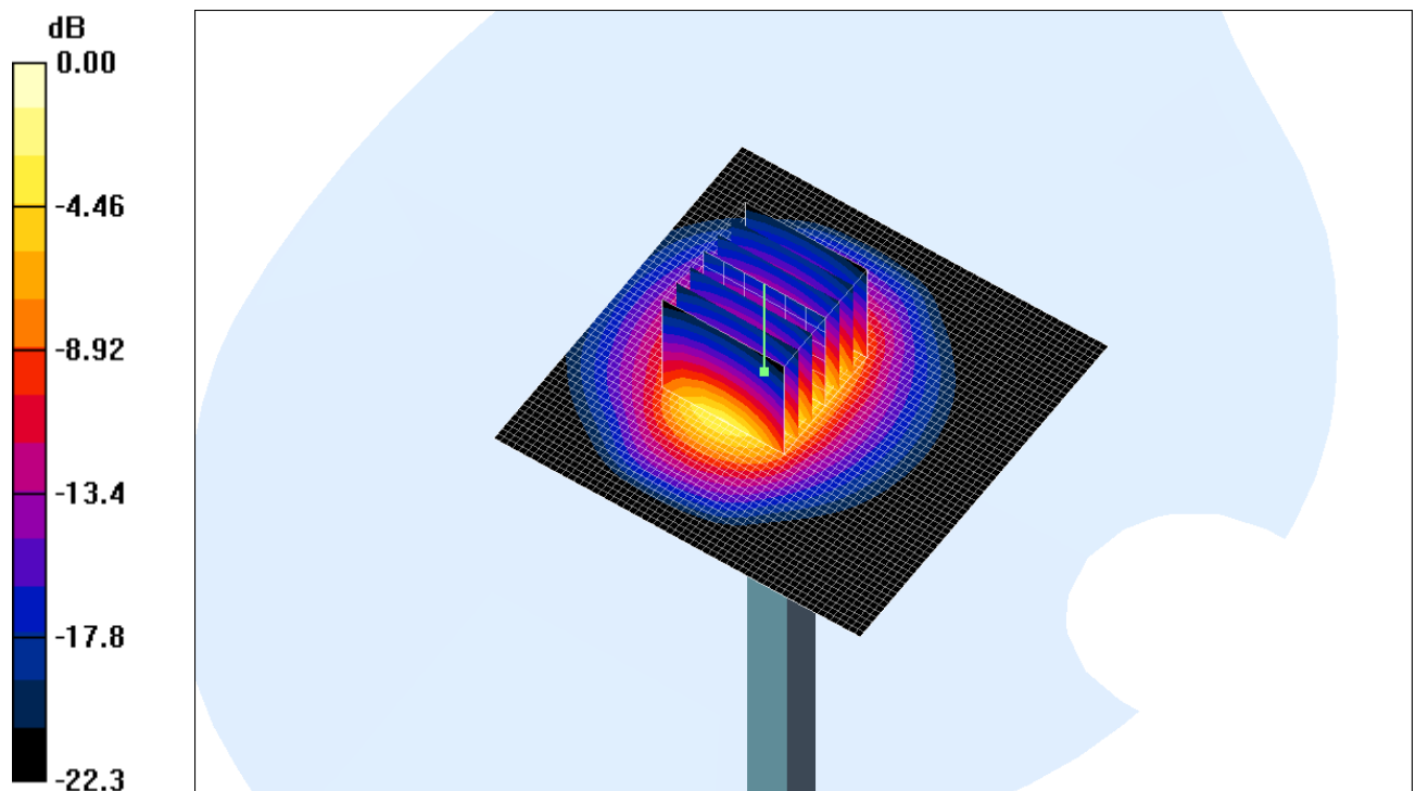
Fig. 7: Résultat de la validation à 2450MHz
