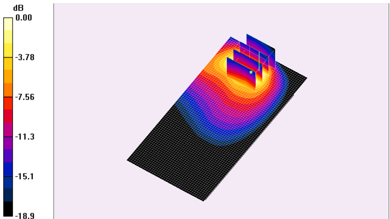
Fig. 16: Distribution du DAS en LTE 800: canal 24300 (847.0 MHz) face arrière à 0cm du fantôme
