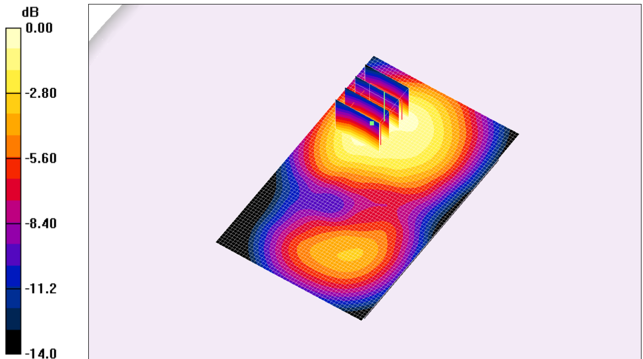
Fig. 11: Distribution du DAS en GSM-GPRS 1800: canal 699 (1747.6 MHz) face arrière à 1.5cm du fantôme
