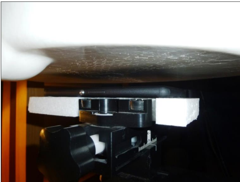
Fig. 25: Face arrière à 1.5cm des fantômes ELI4 et SAM
