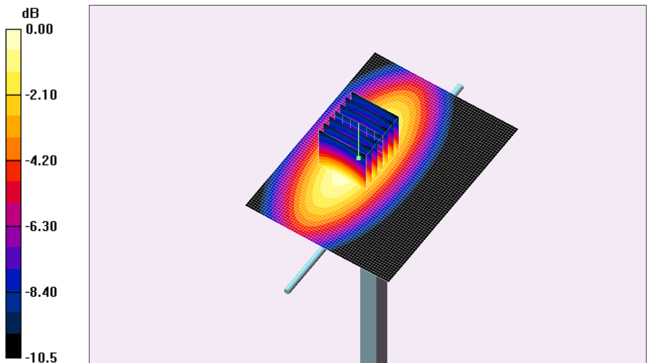
Fig. 3: Résultat de la validation à 835MHz
