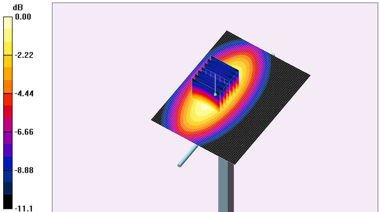
Fig. 4: Résultat de la validation à 900MHz
