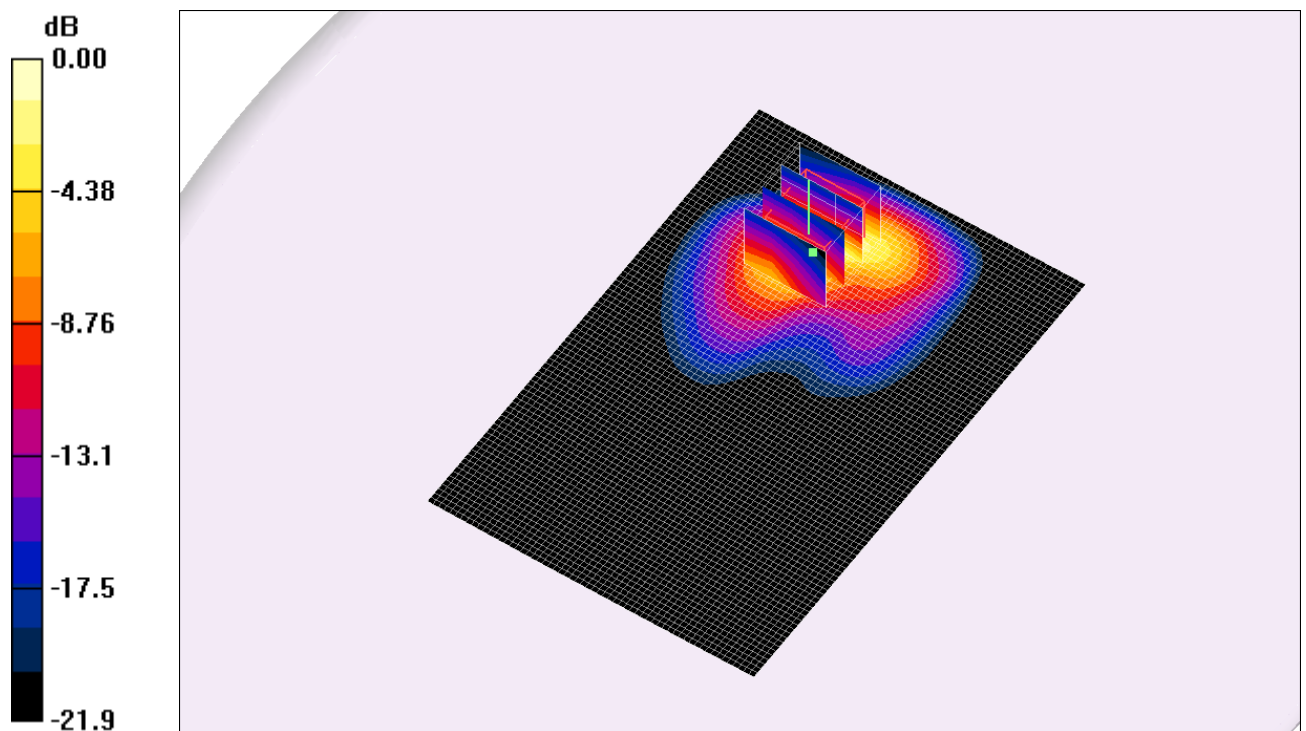
Fig. 14: Distribution du DAS en WCDMA 2100: canal 9750 (1950.0 MHz) face arrière à 0cm du fantôme
