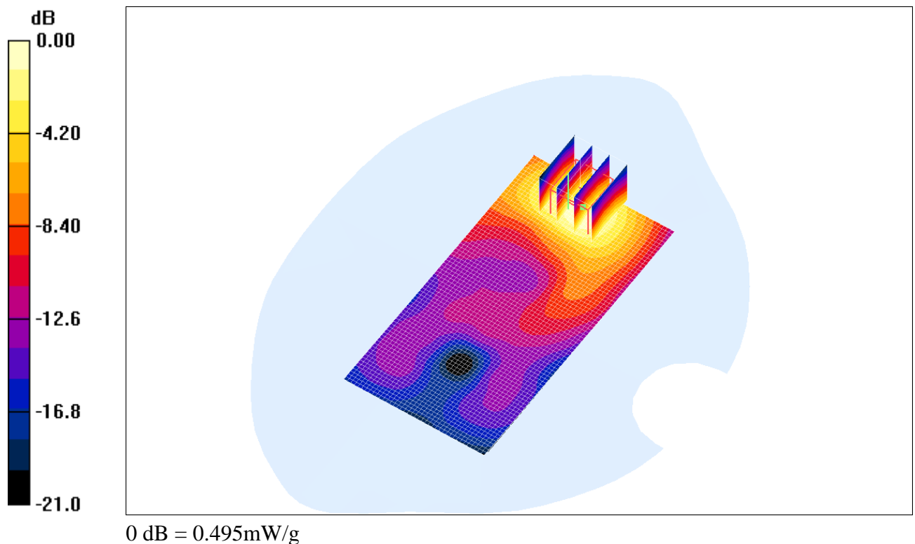
Fig. 22: Distribution du DAS en LTE 2600: canal 21100 (2535.0 MHz) face arrière à 1.5cm du fantôme
