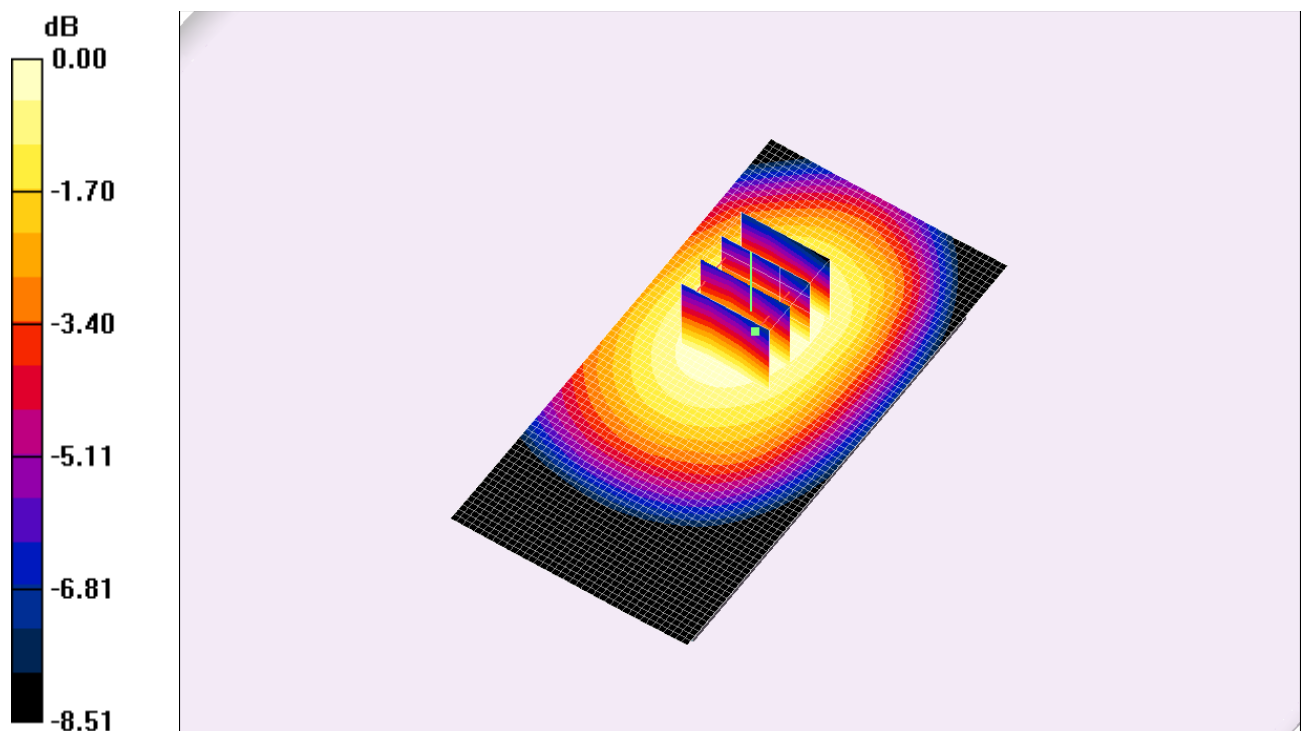
Fig. 17: Distribution du DAS en LTE 800: canal 24300 (847.0 MHz) face arrière à 1.5cm du fantôme
