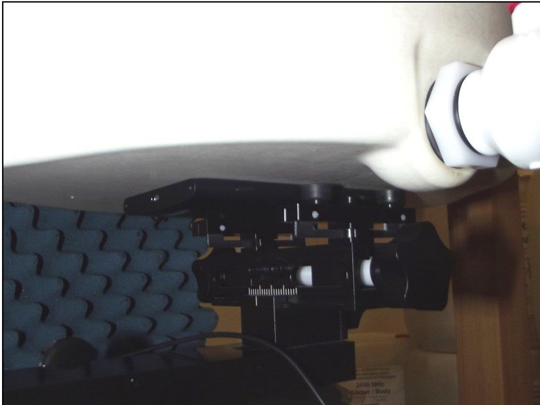
Photo 5: Position d'essai face avant contre le corps (distance 0 mm)
