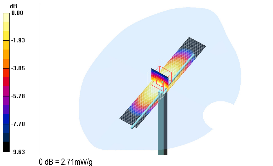
Fig. 3: Résultat de la vérification à 835MHz
