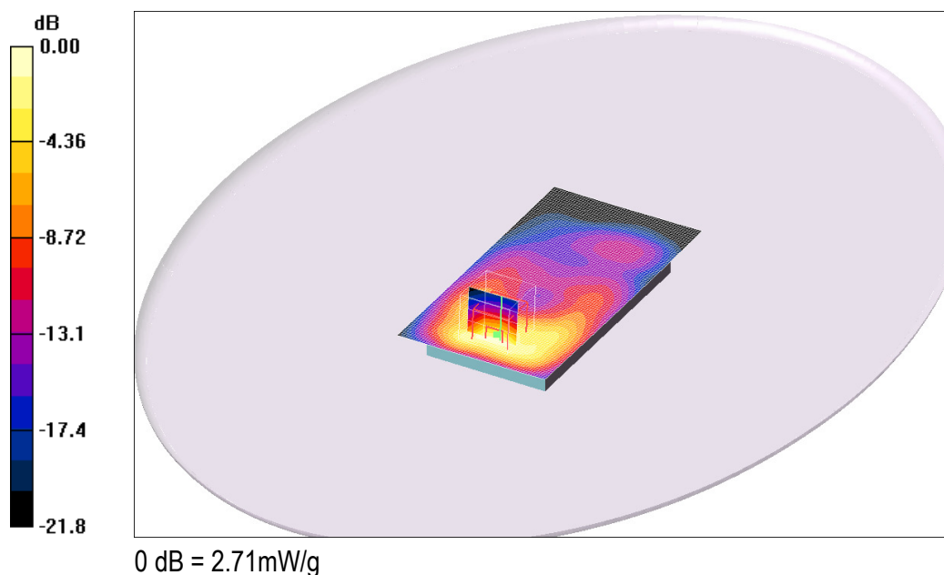
Fig. 14: canal 21425 (2567.5 MHz) – face avant - 5mm
