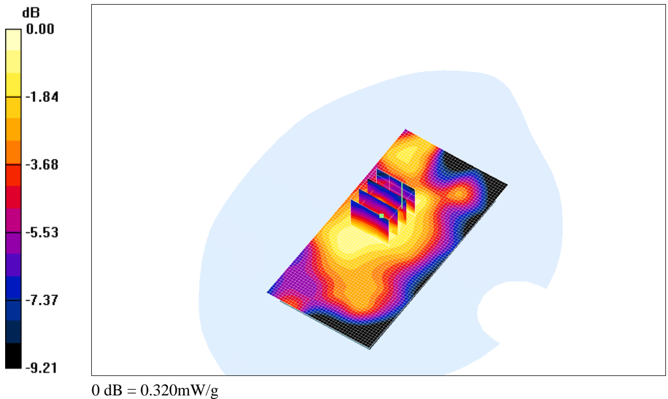
Fig. 10 : Distribution du DAS en WCDMA 900: canal 2712 (882.4 MHz) face arrière à 1.5cm du fantôme
