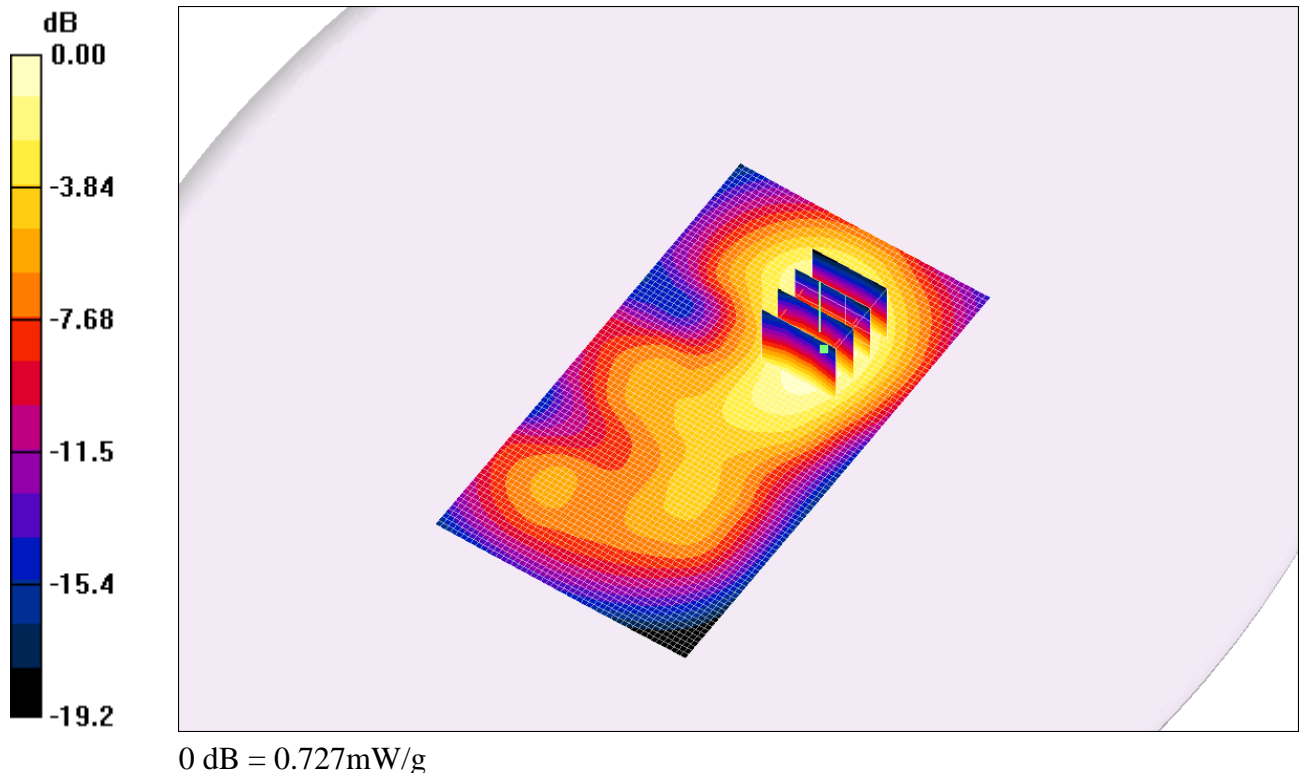
Fig. 14 : Distribution du DAS en LTE 2600: canal 21350 (2560.0 MHz) face avant à 1.5cm du fantôme
