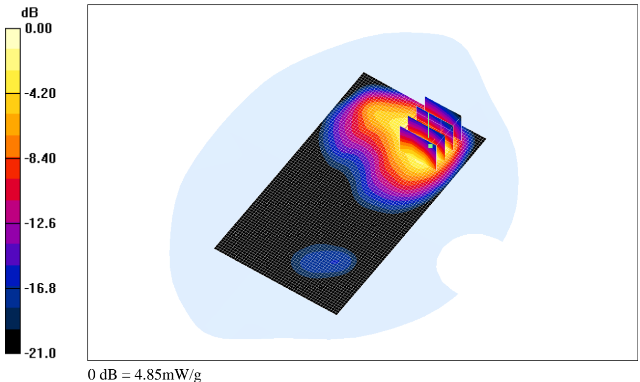
Fig. 13: Distribution du DAS en LTE 1800: canal 19575 (1747.5 MHz) face avant à 0cm du fantôme
