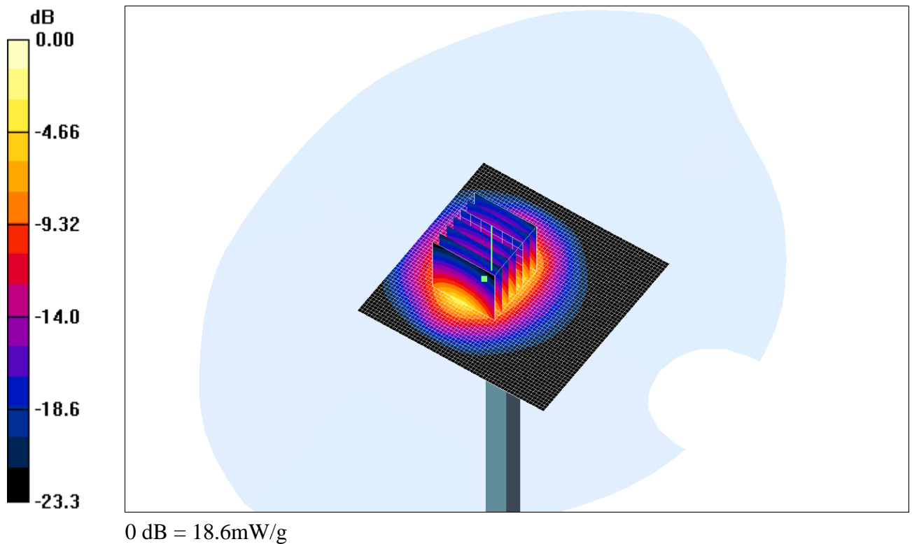
Fig. 7: Résultat de la vérification à 2450MHz
