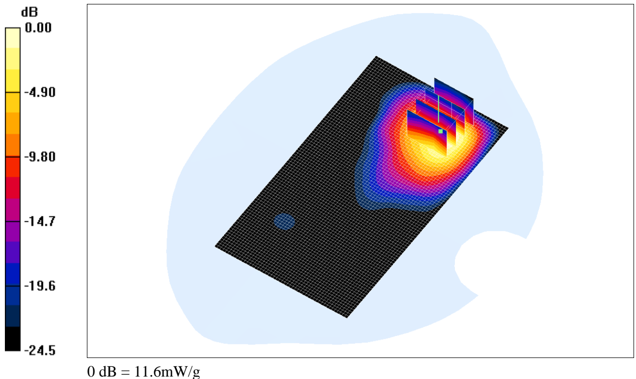
Fig. 14: Distribution du DAS en LTE 2600: canal 21100 (2535.0 MHz) face avant à 0cm du fantôme
