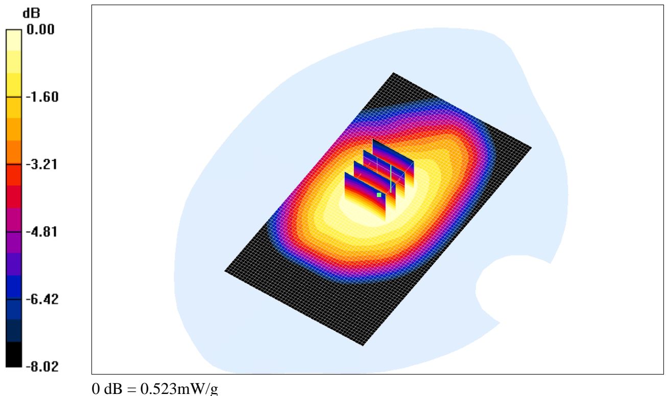
Fig. 10 : Distribution du DAS en WCDMA 900: canal 2788 (897.6 MHz) face avant à 1.5cm du fantôme
