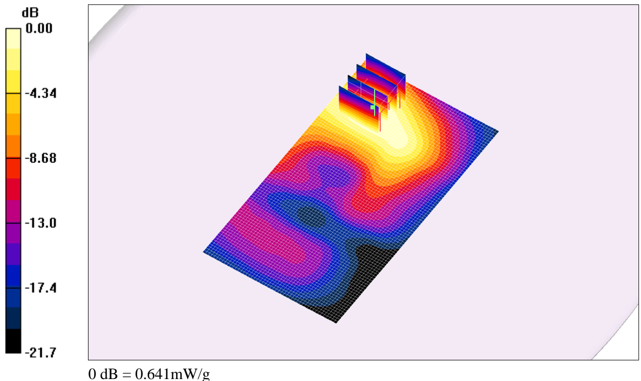
Fig. 14 : Distribution du DAS en LTE 2600: canal 21425 (2567.5 MHz) face arrière à 1.5cm du fantôme
