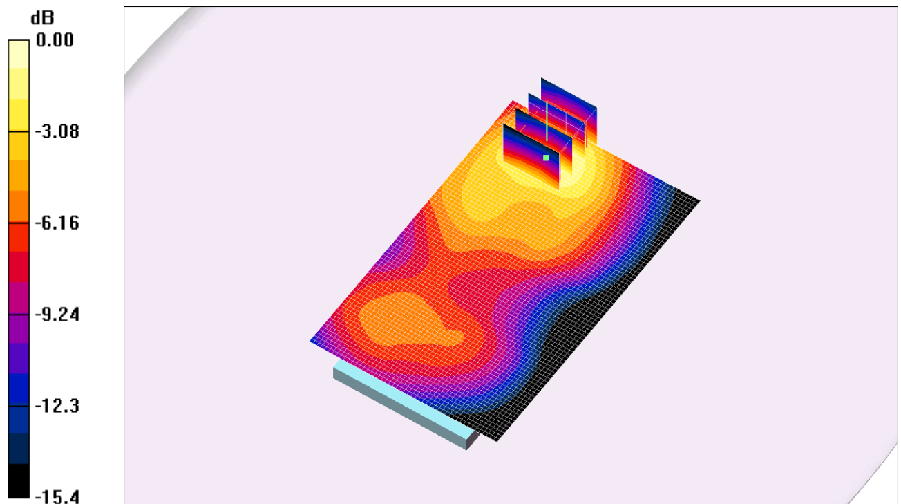
Fig. 9 : Distribution du DAS en GSM-GPRS 1800: canal 885 (1784.8 MHz) face avant à 1.5cm du fantôme
