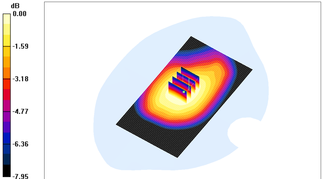
Fig. 8 : Distribution du DAS en GSM-GPRS 900: canal 124 (914.8 MHz) face avant à 1.5cm du fantôme
