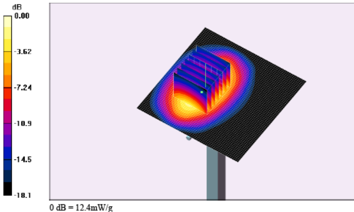
Fig. 5: Résultat de la vérification à 1800MHz
