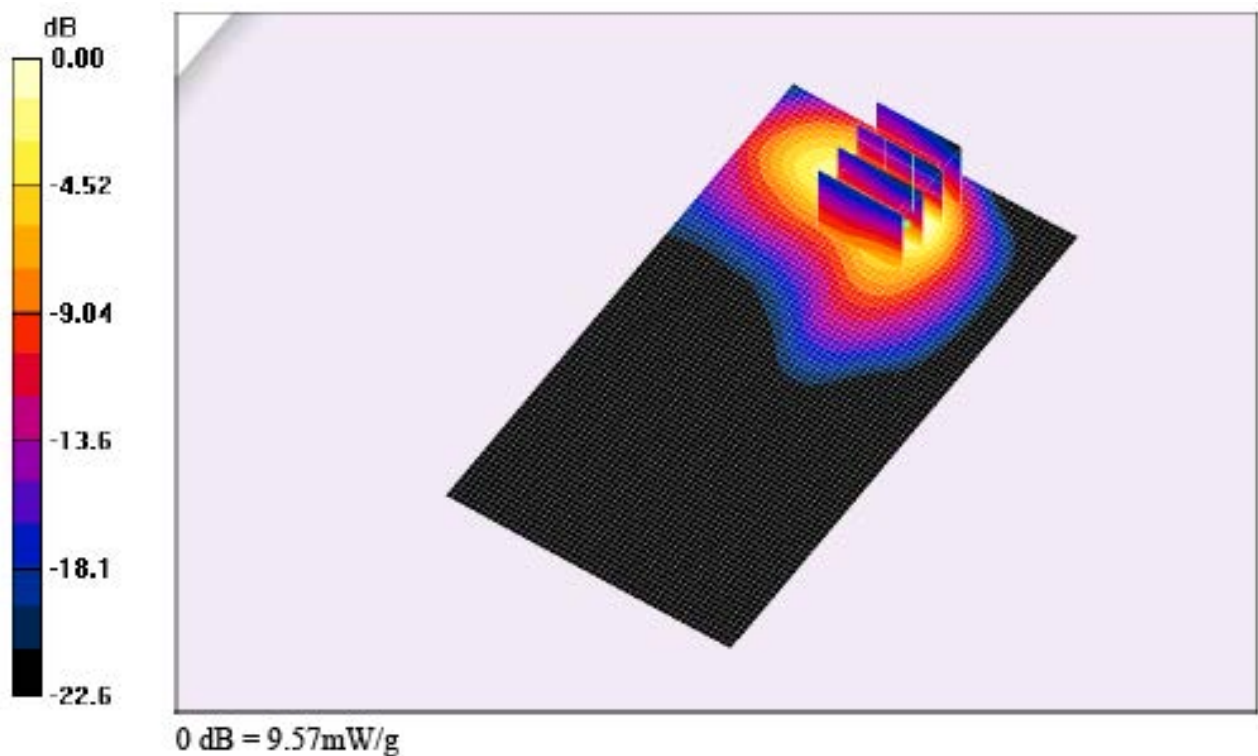
Fig. 9: Distribution du DAS en GSM-GPRS 1800: canal 885 (1784.8 MHz) face avant à 0cm du fantôme
