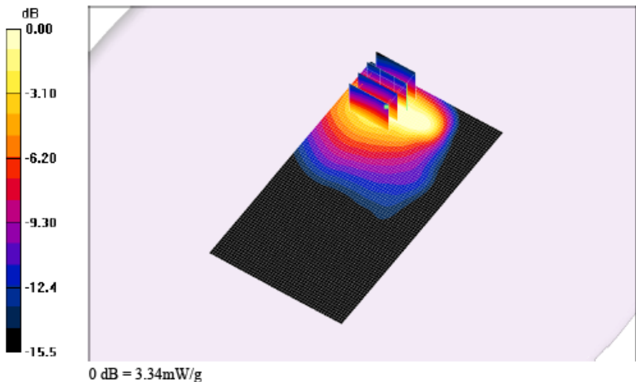
Fig. 12: Distribution du DAS en LTE 800: canal 24250 (842.0 MHz) face arrière à 0cm du fantôme
