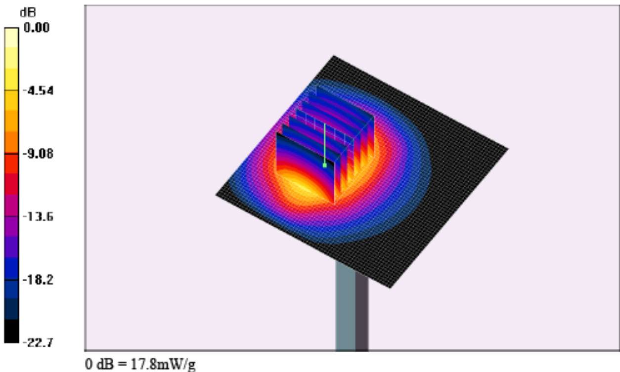
Fig. 7 : Résultat de la vérification à 2450MHz
