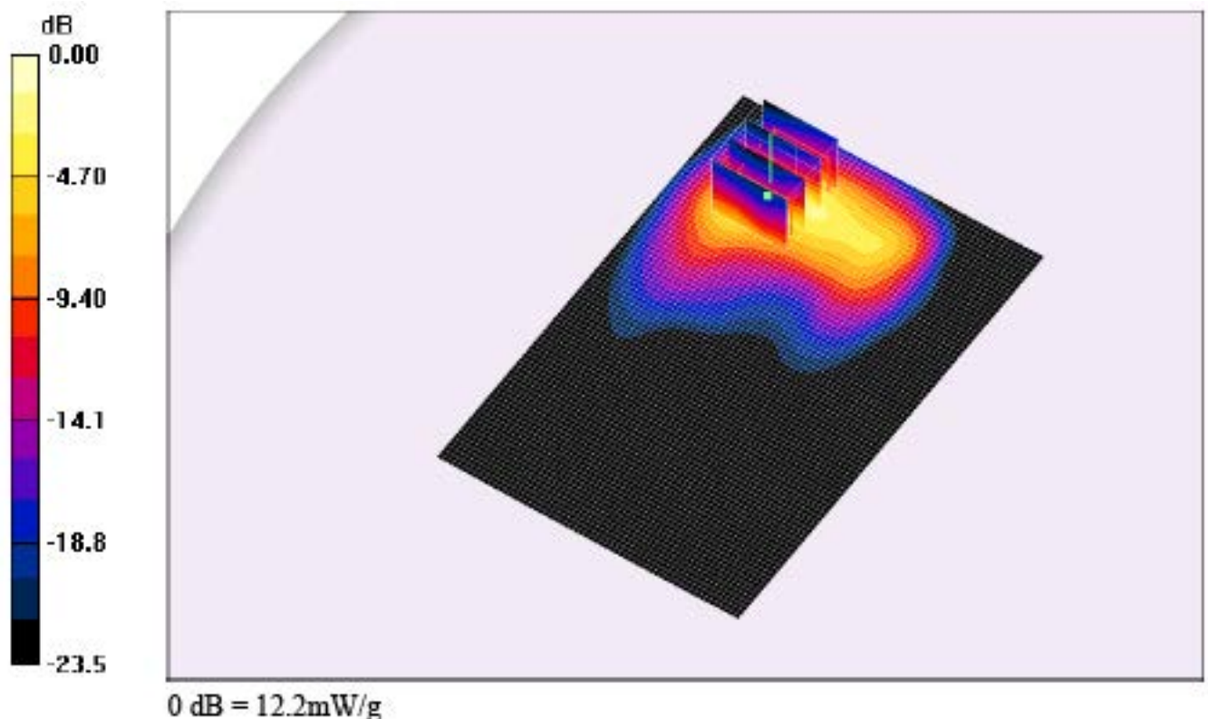
Fig. 13: Distribution du DAS en LTE 1800: canal 19943 (1784.3 MHz) face arrière à 0cm du fantôme
