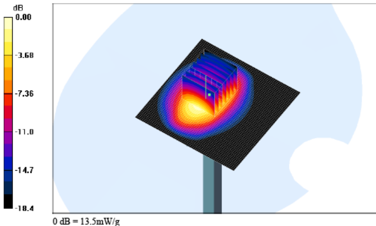
Fig. 6: Résultat de la vérification à 1950MHz
