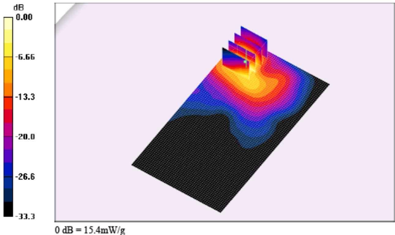
Fig. 14: Distribution du DAS en LTE 2600: canal 21100 (2535.0 MHz) face arrière à 0cm du fantôme
