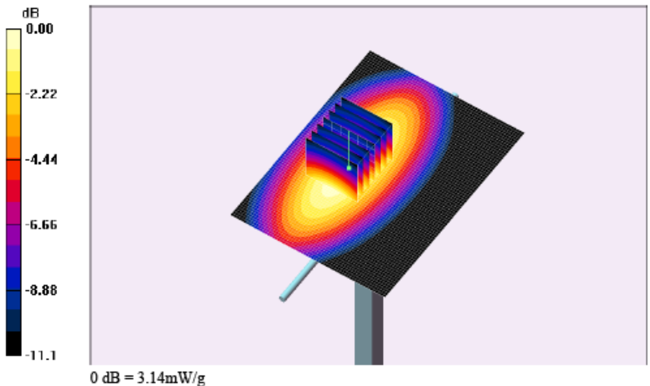
Fig. 4: Résultat de la vérification à 900MHz
