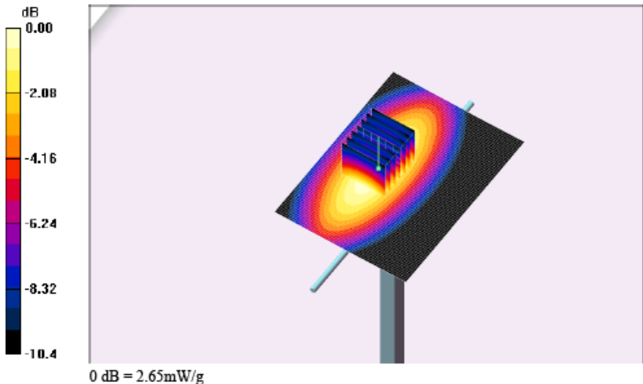
Fig. 3: Résultat de la vérification à 835MHz
