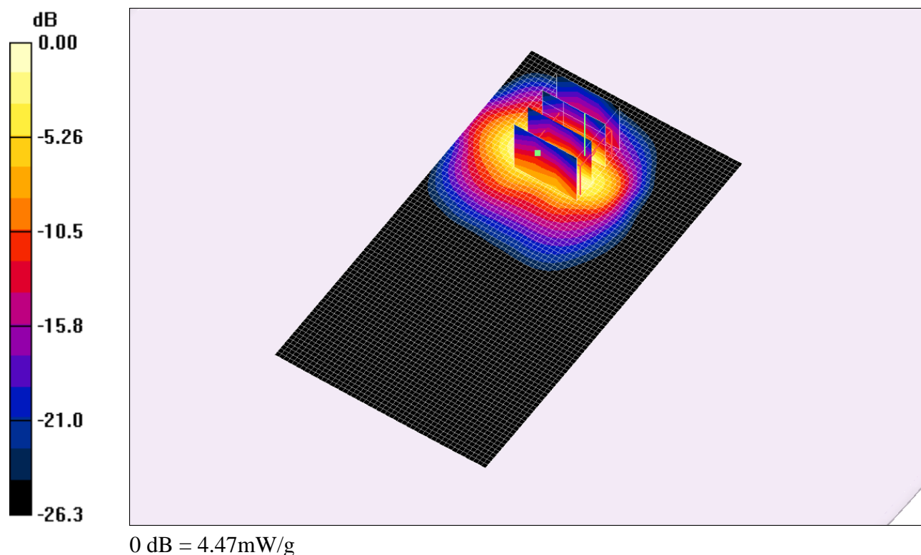
Fig. 14: Distribution du DAS en LTE 2600: canal 20775 (2502.5 MHz) face arrière à 0cm du fantôme
