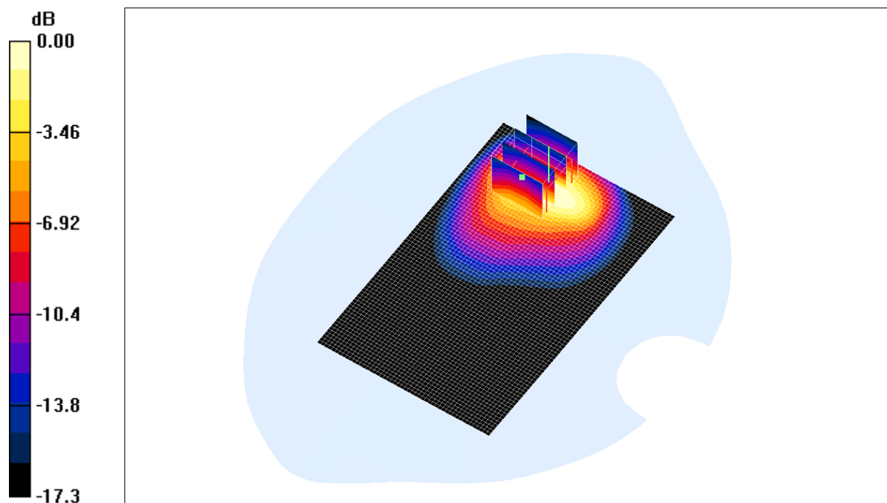
Fig. 10: Distribution du DAS en WCDMA 900: canal 2712 (882.4 MHz) face arrière à 0cm du fantôme
