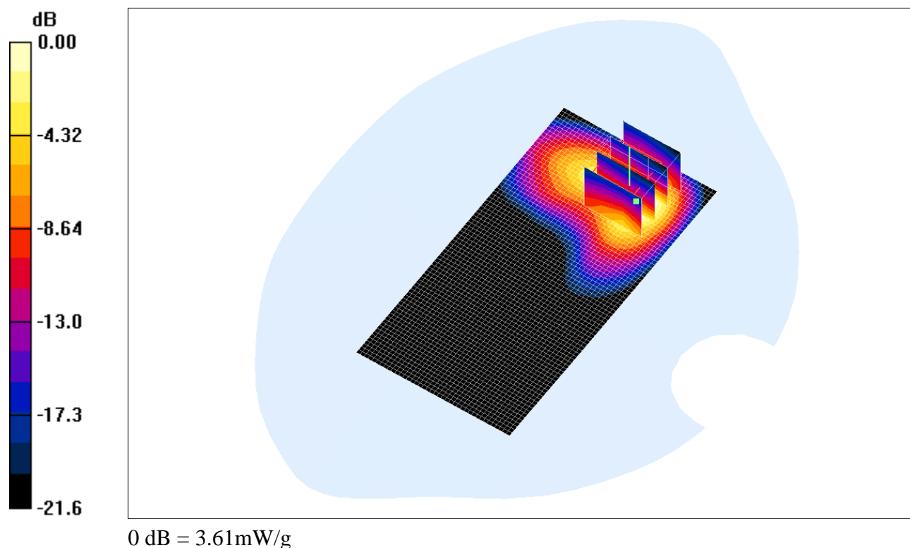
Fig. 11: Distribution du DAS en WCDMA 2100: canal 9888 (1977.6 MHz) face arrière à 0cm du fantôme
