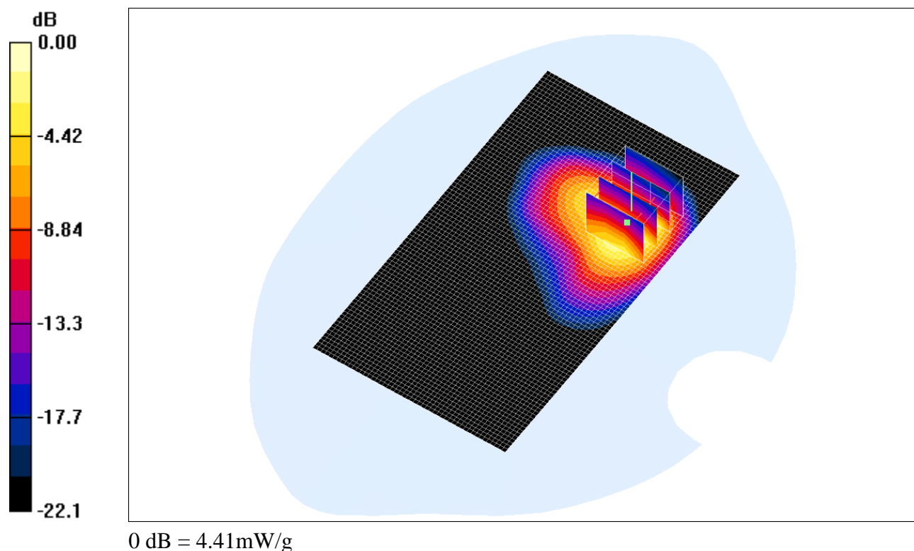
Fig. 13: Distribution du DAS en LTE 1800: canal 19300 (1720.0 MHz) face arrière à 0cm du fantôme
