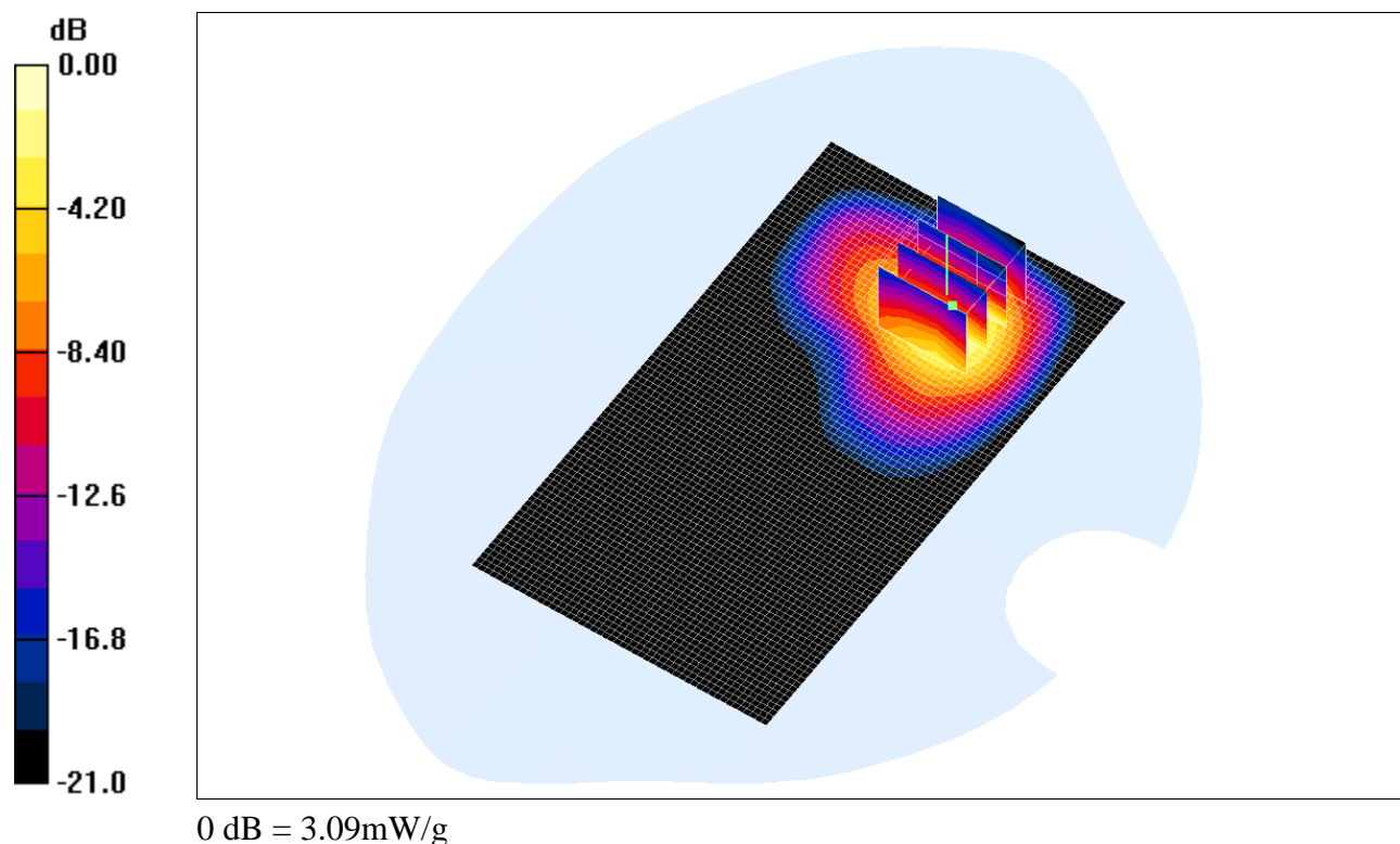
Fig. 9: Distribution du DAS en GSM-GPRS 1800: canal 512 (1710.2 MHz) face arrière à 0cm du fantôme
