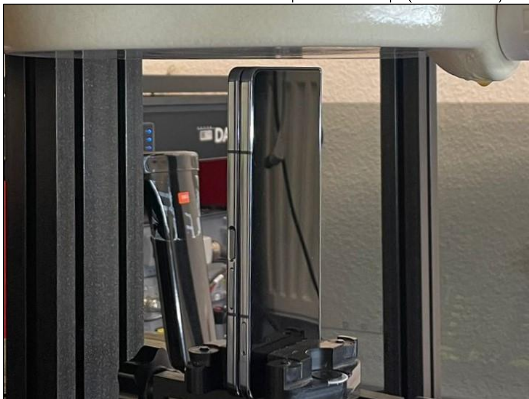
Photo 16: Position d'essai face du dessous plié contre le corps (distance 5 mm)
