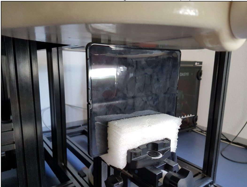
Photo 9: Position d'essai face du côté gauche contre le corps (distance 5 mm)
