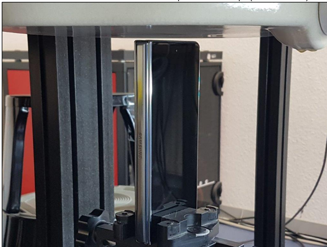
Photo 15: Position d'essai face du dessus plié contre le corps (distance 5 mm)
