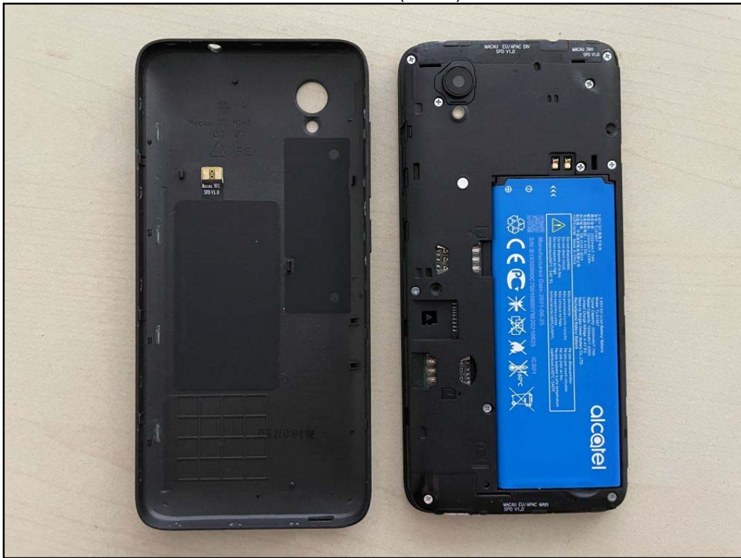
Photo 6: EST – vue arrière (ouvert) avec batterie
