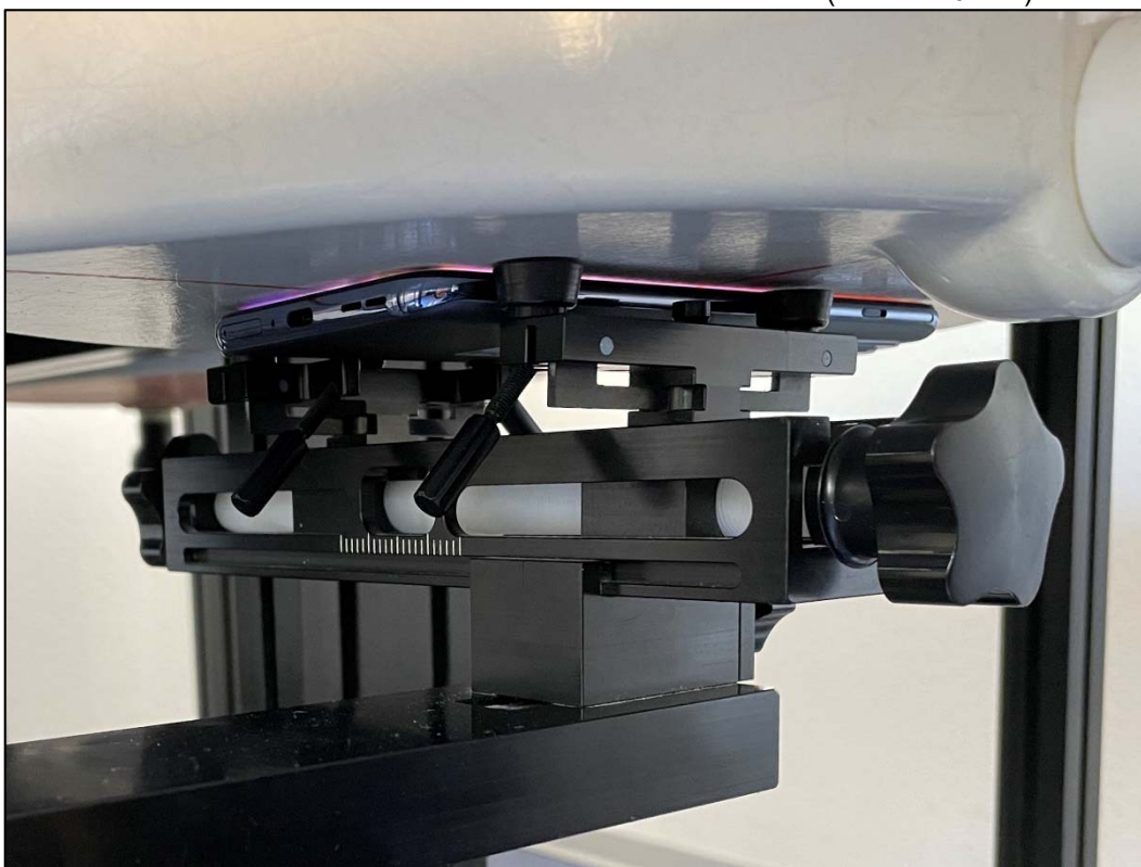
Photo 8: Position d'essai face arrière contre le membre (distance 0 mm)
