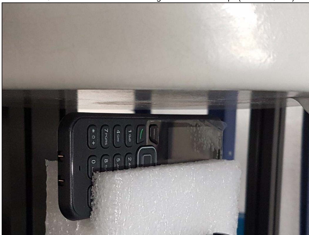
Photo 11: Position d'essai face du côté droite contre le corps (distance 5 mm)
