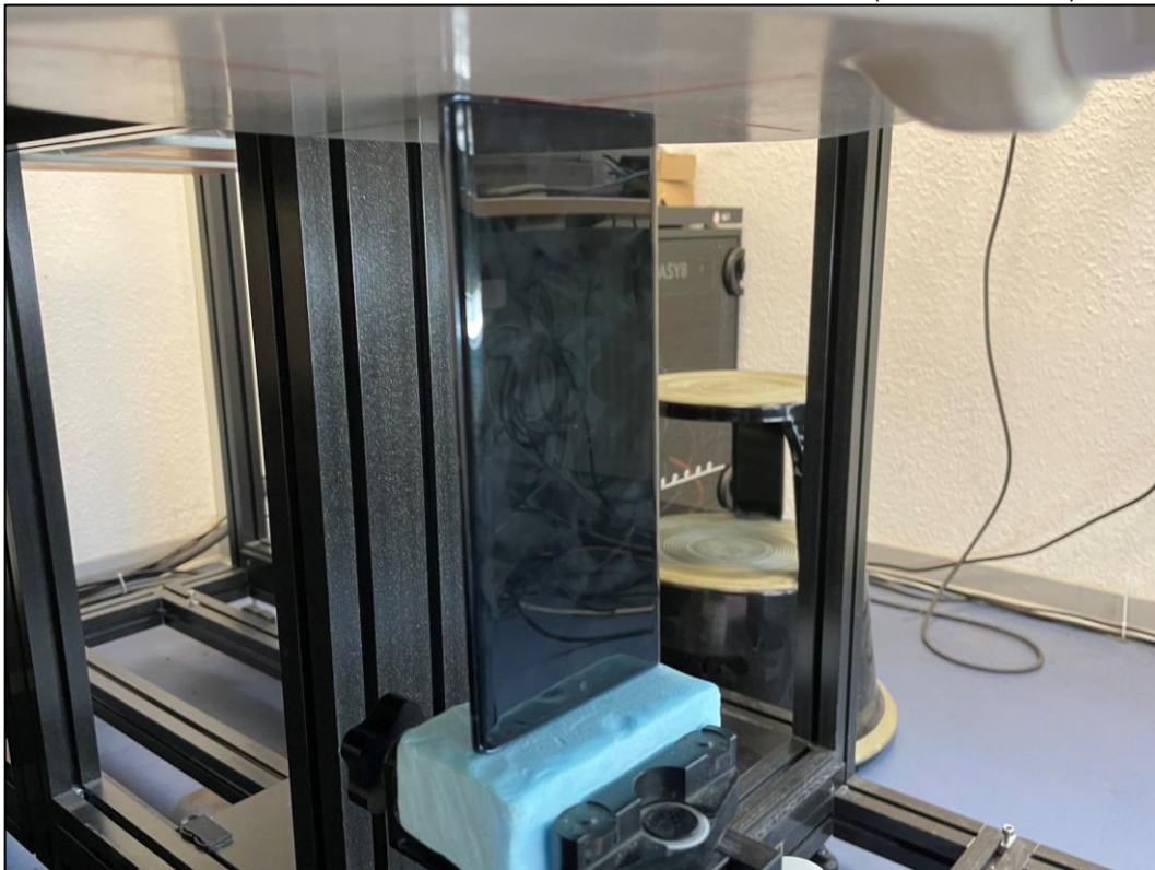
Photo 7: Position d'essai face du dessous contre le membre (distance 0 mm)
