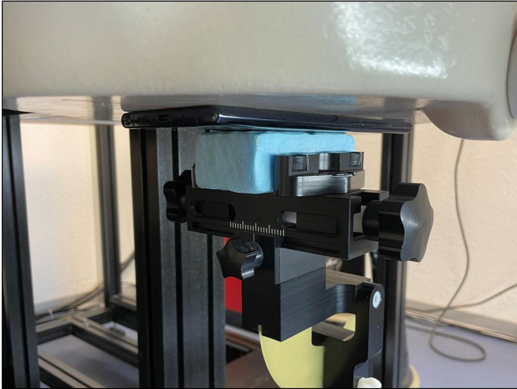
Photo 6: Position d'essai face arrière contre le membre (distance 0 mm)
