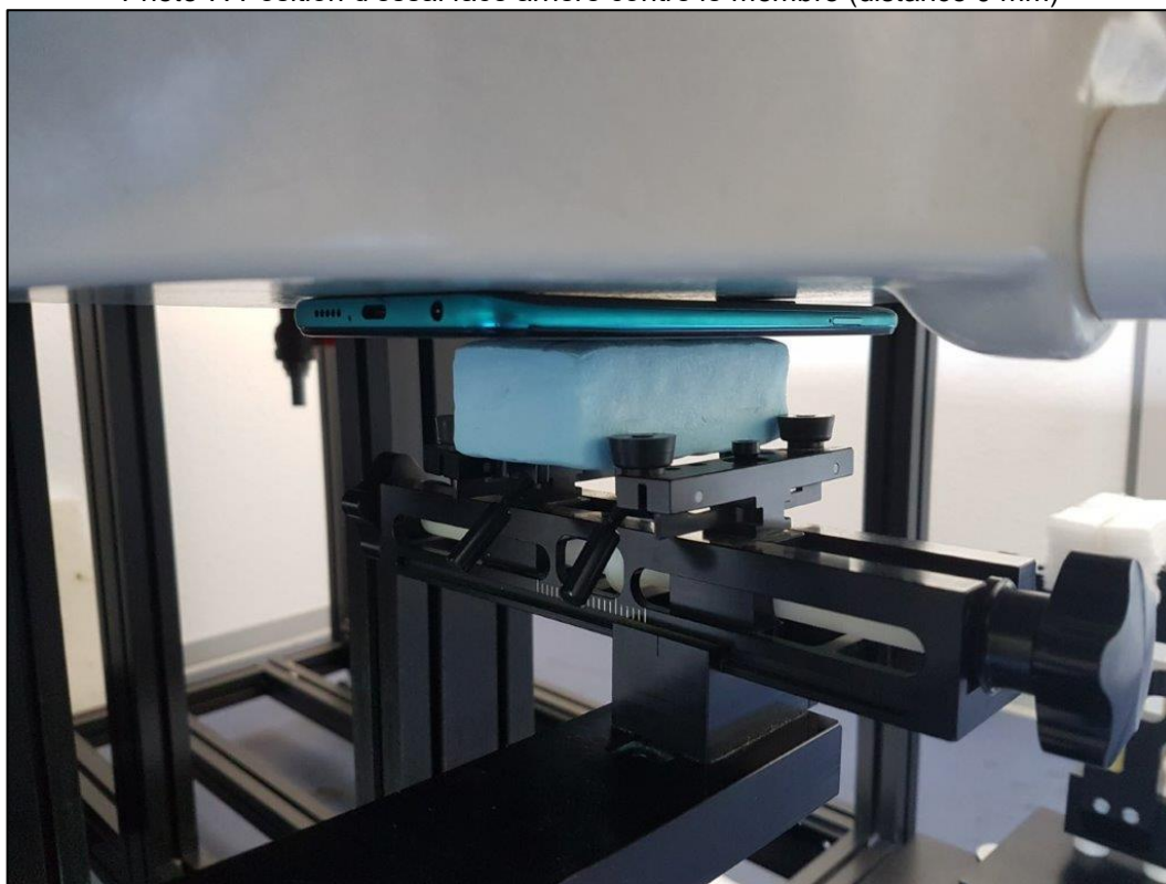
Photo 8: Position d'essai face du dessous contre le membre (distance 0 mm)
