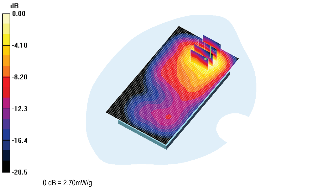
Fig. 13: Distribution du DAS en LTE 1800: canal 19575 (1747.5 MHz) face arrière à 0.5cm du fantôme
