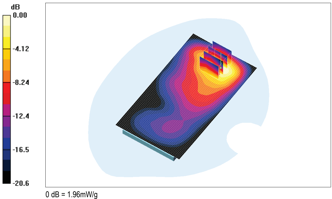
Fig. 9: Distribution du DAS en GSM-GPRS 1800: canal 885 (1784.8 MHz) face arrière à 0.5cm du fantôme
