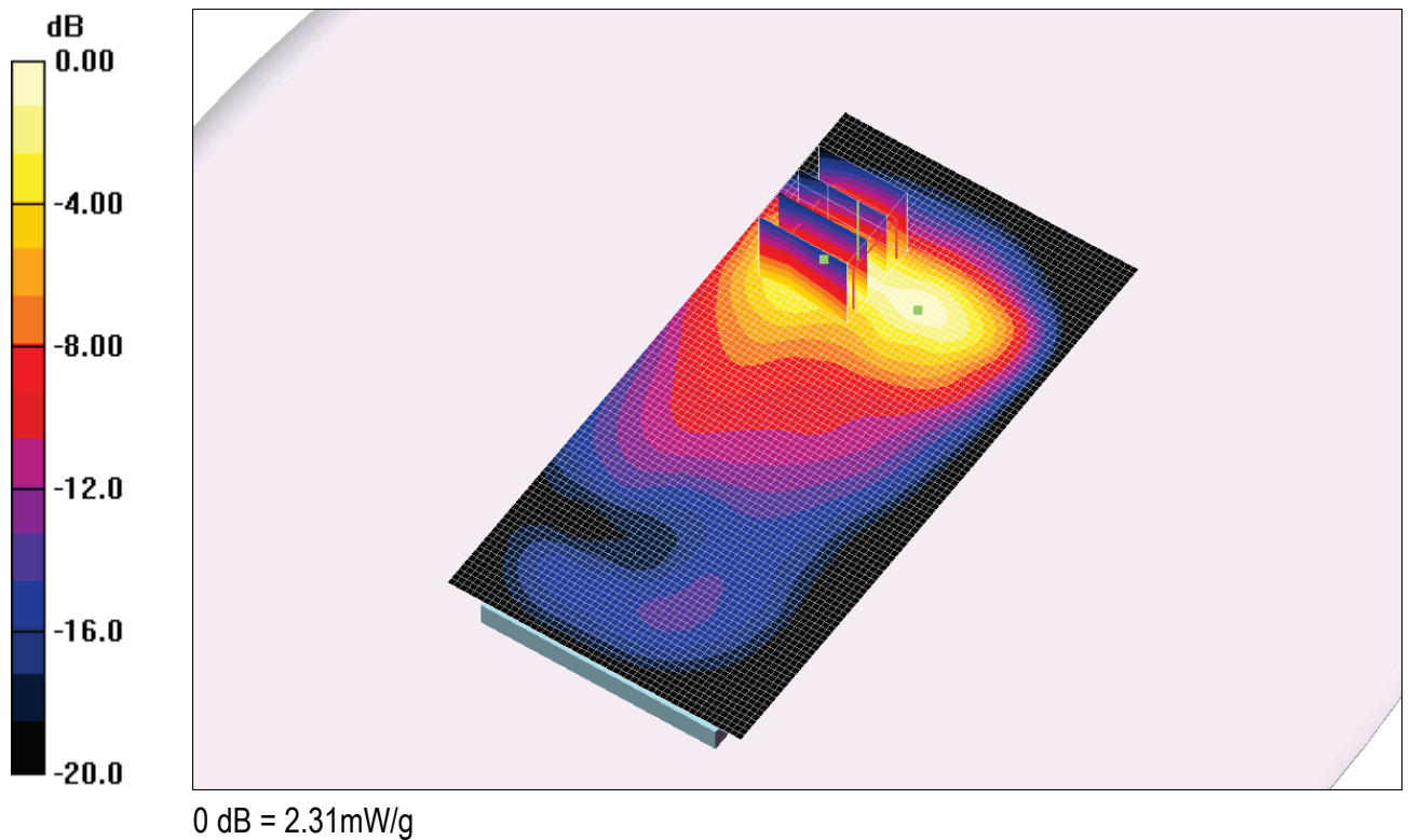
Fig. 11: Distribution du DAS en WCDMA 2100: canal 9750 (1950.0 MHz) face arrière à 0.5cm du fantôme
