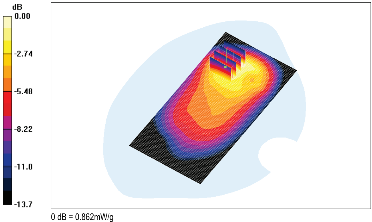
Fig. 12: Distribution du DAS en LTE 800: canal 24425 (859.5 MHz) face arrière à 0.5cm du fantôme
