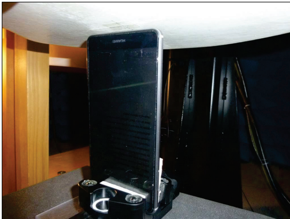
Fig. 20 : Dessous à 0.5cm du fantôme
