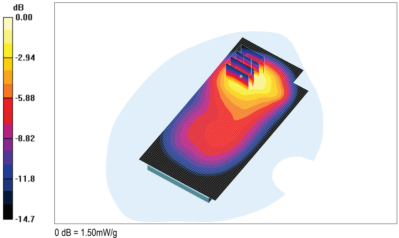
Fig. 8 : Distribution du DAS en GSM-GPRS 900: canal 038 (897.6 MHz) face avant à 0.5cm du fantôme
