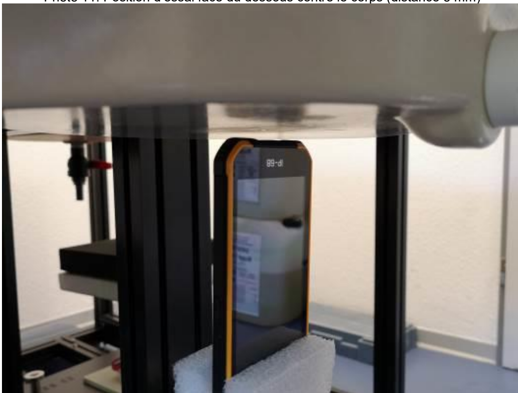
Photo 11: Position d'essai face du dessous contre le corps (distance 5 mm)
