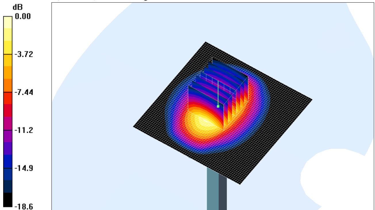
Fig. 5: Résultat de la vérification à 1950MHz
