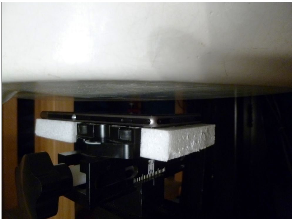
Fig. 17: Face arrière à 1.5cm du fantôme
