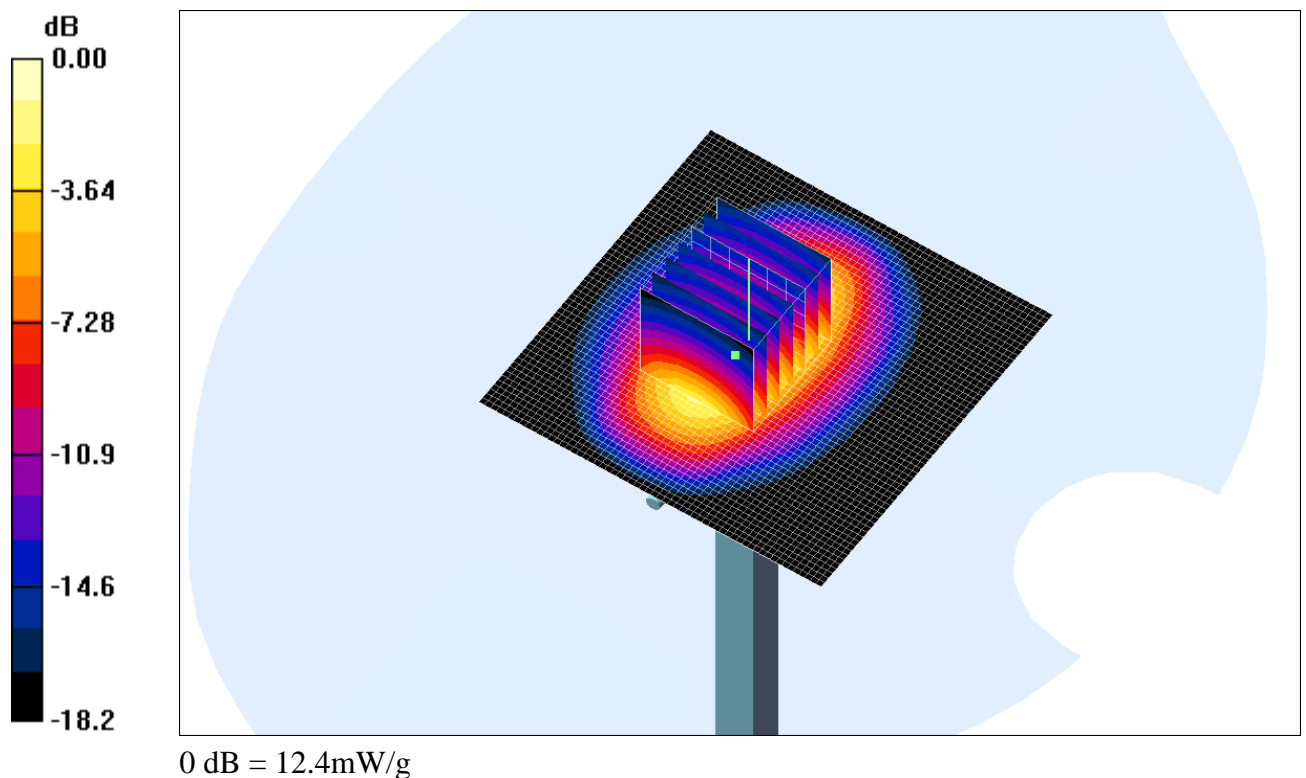
Fig. 4: Résultat de la vérification à 1800MHz
