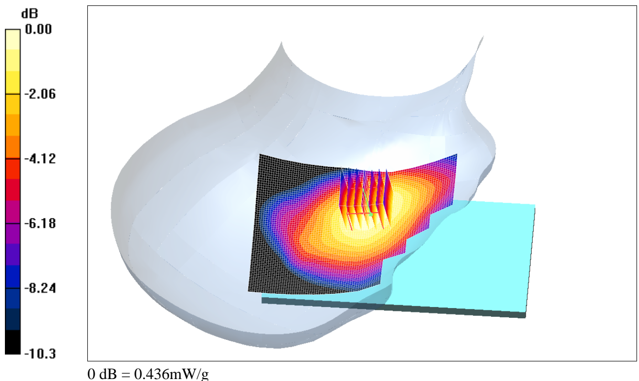
Fig. 6 : Distribution du DAS en GSM900: canal 038 (897.6 MHz), position joue, côté droit
