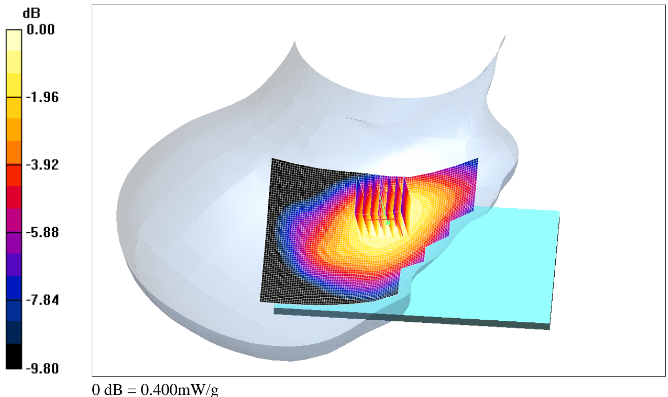
Fig. 8 : Distribution du DAS en WCDMA900: canal 2712 (882.4 MHz), position joue, côté droit
