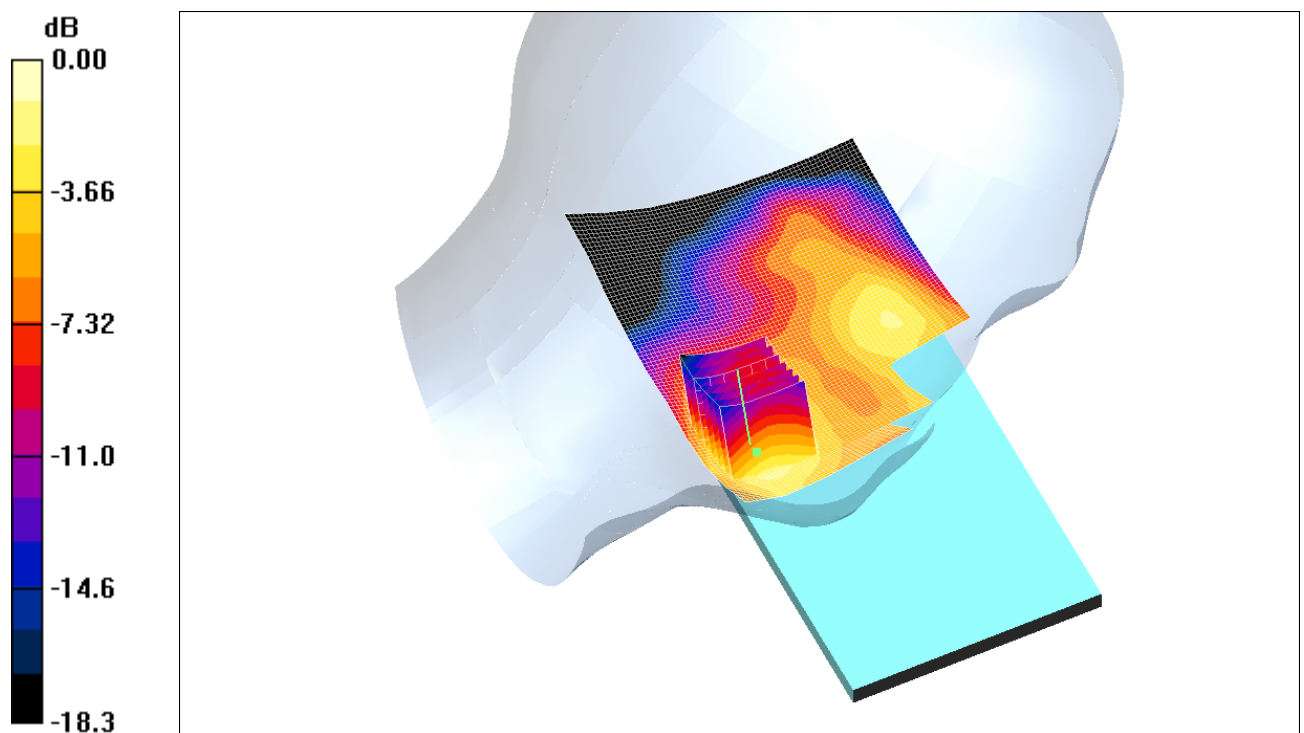
Fig. 7 : Distribution du DAS en GSM1800: canal 512 (1710.2 MHz), position joue, côté gauche
