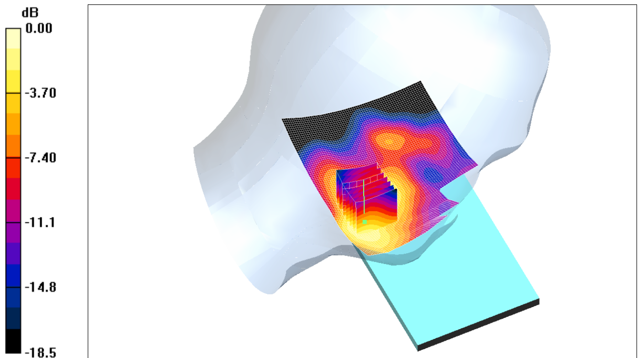
Fig. 9 : Distribution du DAS en WCDMA2100: canal 9888 (1977.6 MHz), position joue, côté gauche
