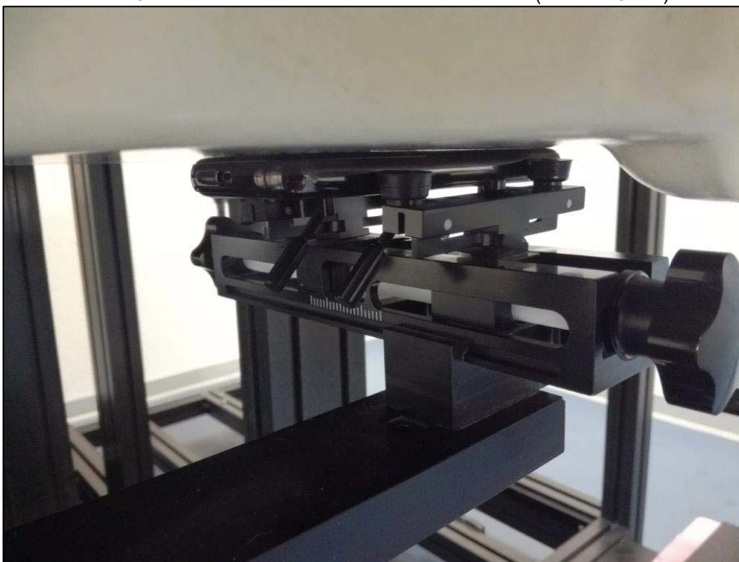
Photo 10: Position d'essai face arrière contre le membre (distance 0 mm)
