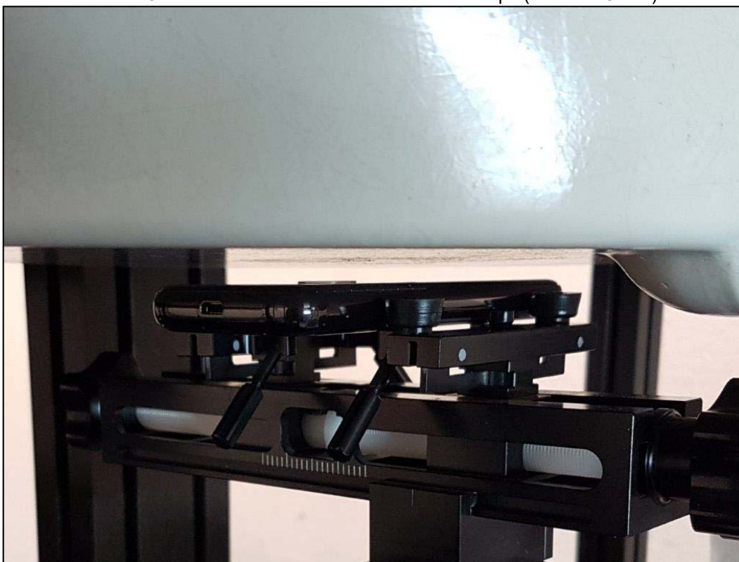
Photo 10: Position d'essai face arrière contre le corps (distance 5 mm)
