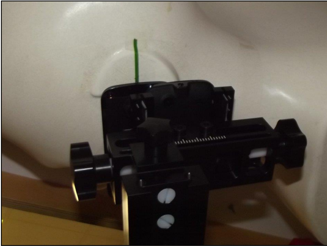
Photo 24: Position d'essai main droite, incliné 15° (glissière ouverte)
