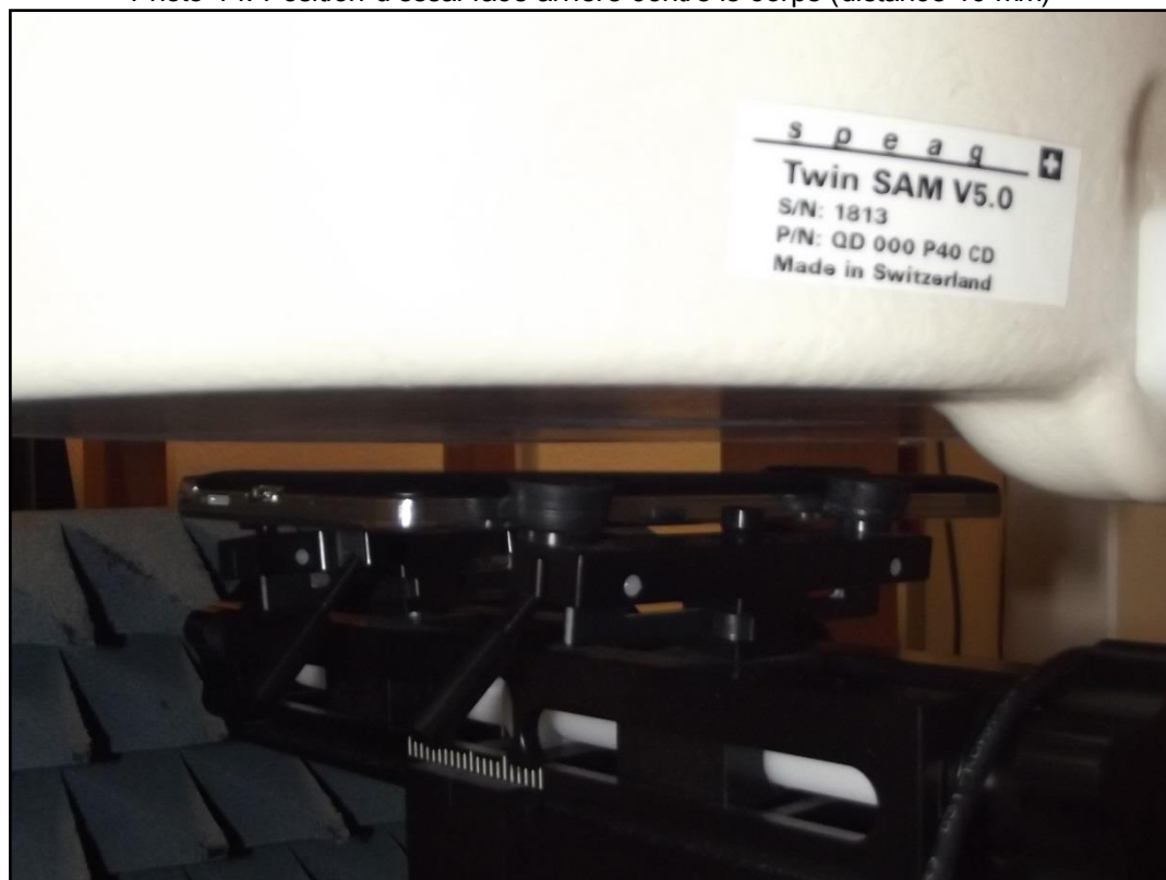
Photo 14: Position d'essai face arrière contre le corps (distance 10 mm)
