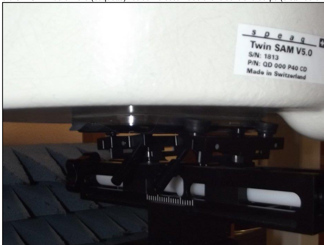
Photo 8: EST – vue arrière (étiquette) Position d'essai face avant contre le corps (distance 0 mm)
