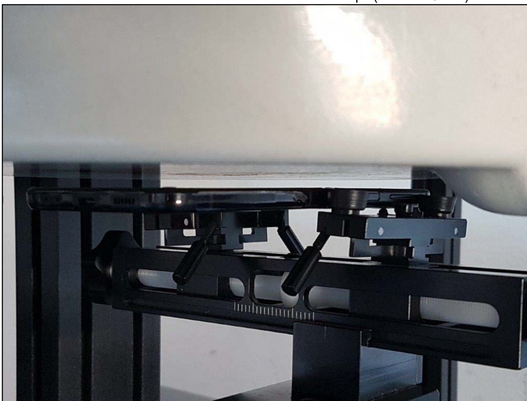
Photo 8: Position d'essai face arrière contre le corps (distance 5 mm)
