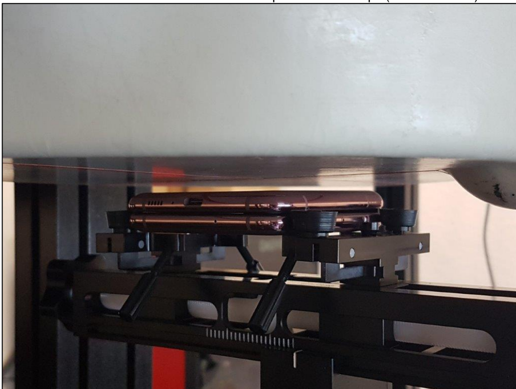
Photo 14: : Position d'essai face arrière pliée contre le corps (distance 5 mm)
