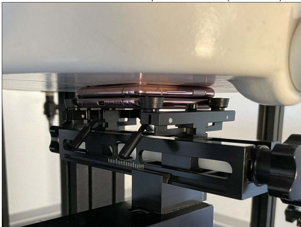
Photo 14: : Position d'essai face arrière pliée contre le membre (distance 0 mm)
