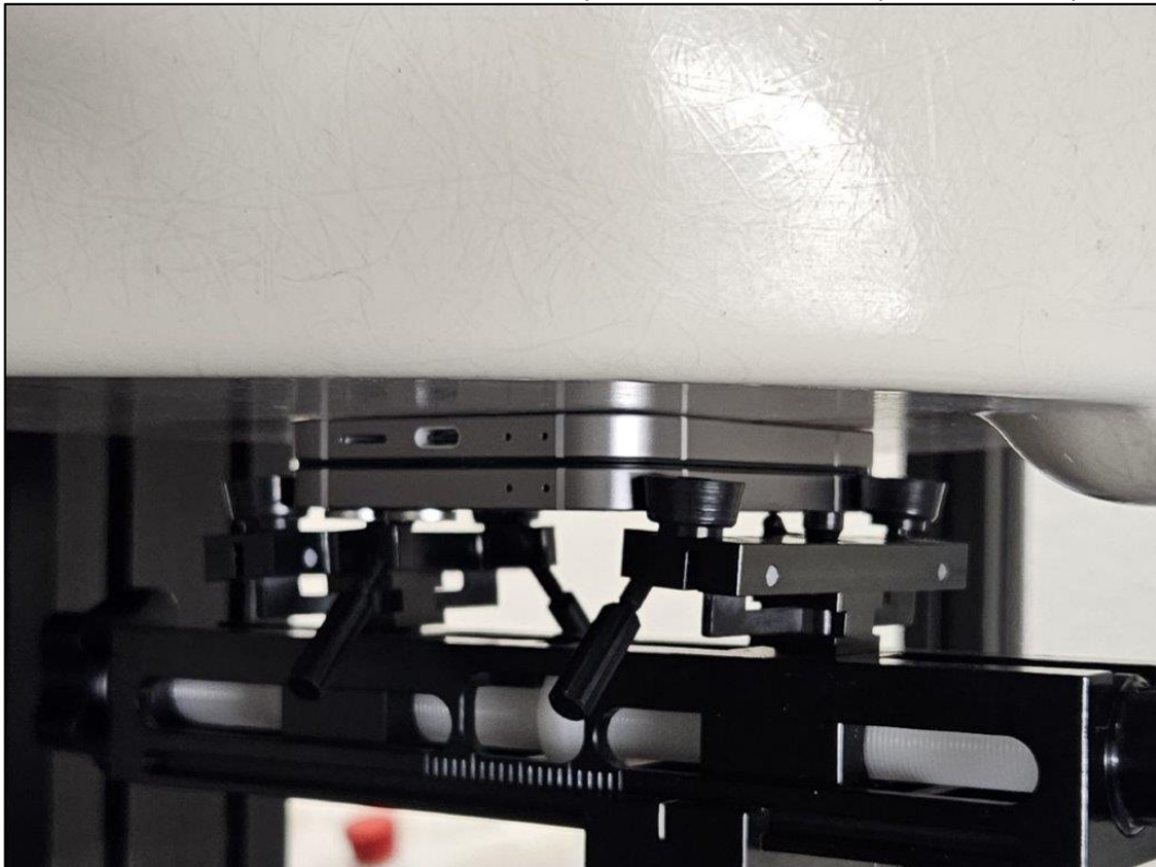
Photo 14: Position d'essai face arrière pilé contre le membre (distance 0 mm)
