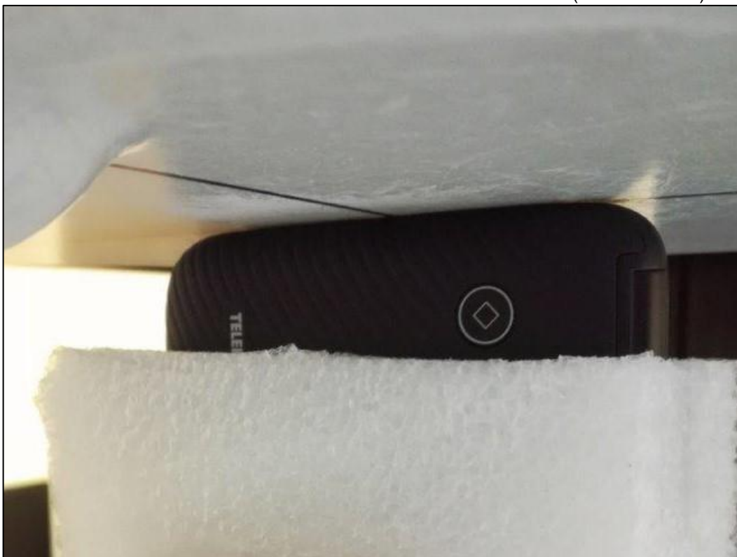
Photo 14: Position d'essai face du côté droite contre le membre (distance 0 mm)
