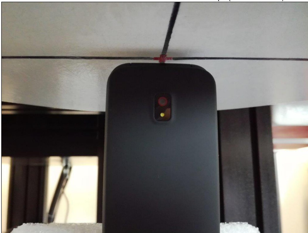
Photo 15: Position d'essai face du dessus contre le corps (distance 5 mm)
