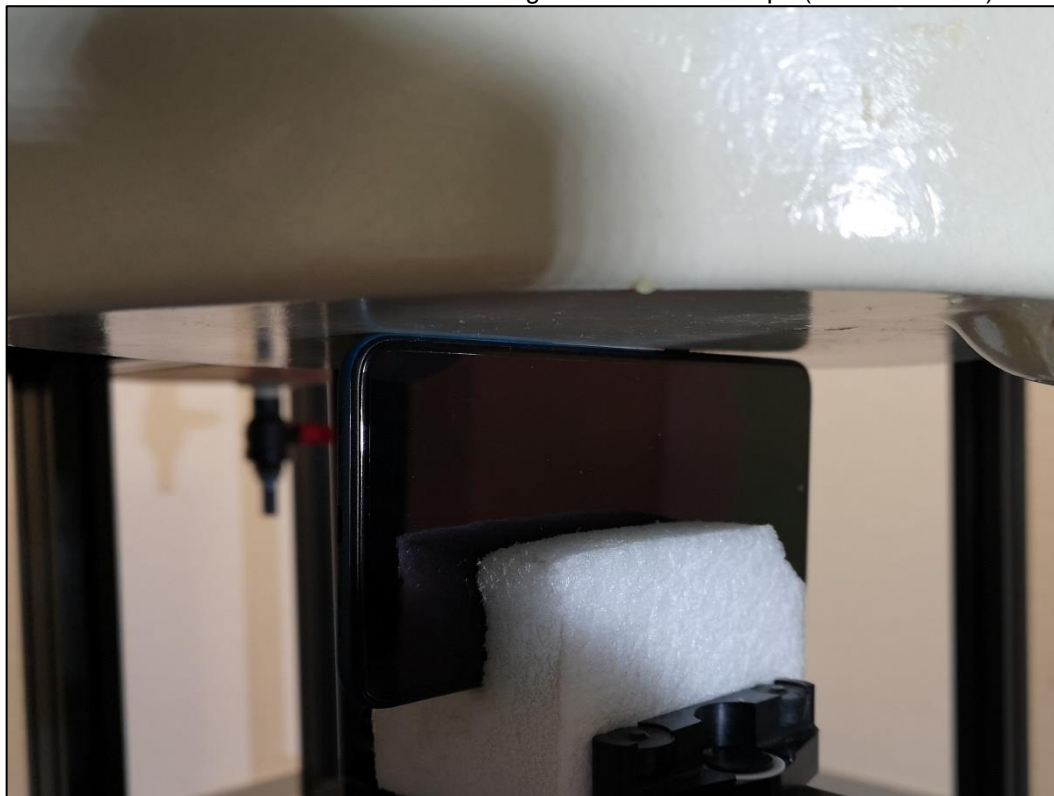
Photo 9: Position d'essai face du côté gauche contre le corps (distance 0 mm)
