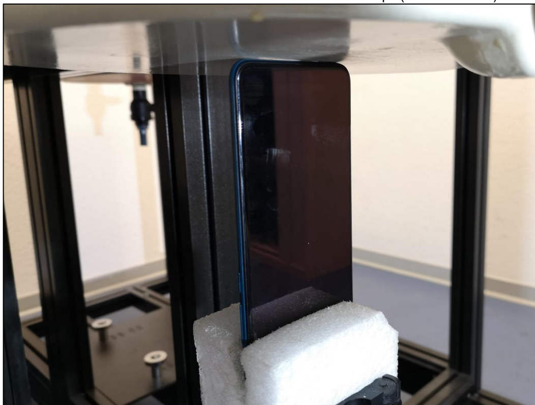
Photo 12: Position d'essai face du dessous contre le corps (distance 0 mm)
