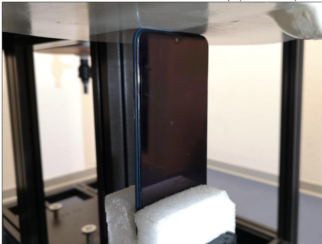
Photo 11: Position d'essai face du dessus contre le corps (distance 0 mm)
