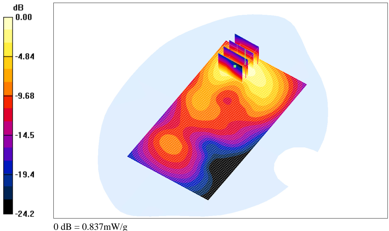
Fig. 14 : Distribution du DAS en LTE 2600: canal 21350 (2560.0 MHz) face arrière à 1.5cm du fantôme
