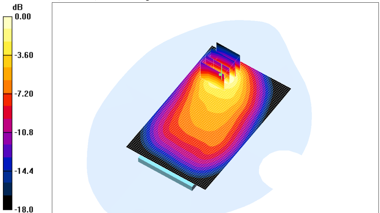
Fig. 8 : Distribution du DAS en GSM-GPRS 900: canal 038 (897.6 MHz) face arrière à 0.5cm du fantôme
