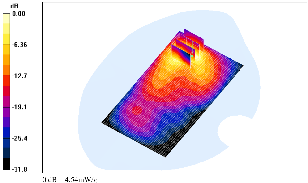
Fig. 14 : Distribution du DAS en LTE 2600: canal 21350 (2560.0 MHz) face arrière à 0.5cm du fantôme
