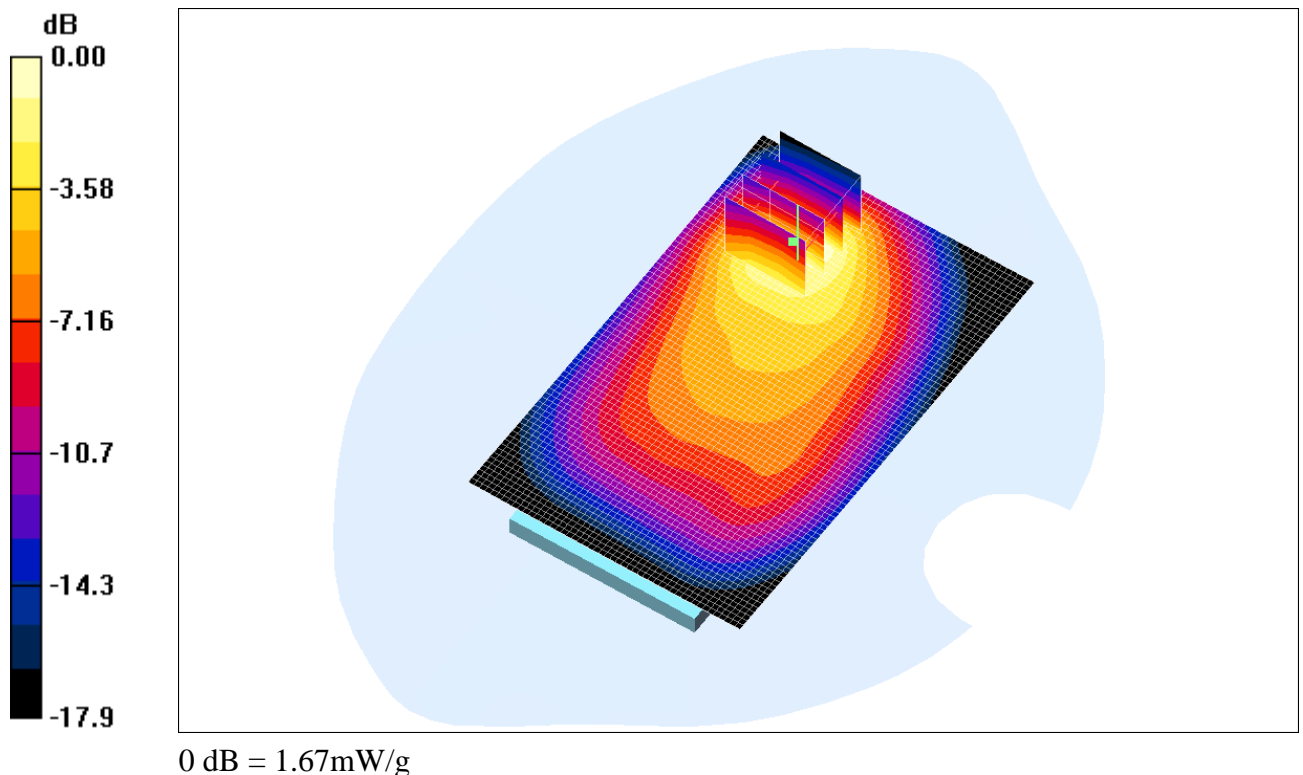
Fig. 10 : Distribution du DAS en WCDMA 900: canal 2788 (897.6 MHz) face arrière à 0.5cm du fantôme
