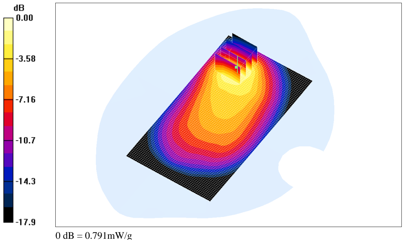
Fig. 12 : Distribution du DAS en LTE 800: canal 24250 (842.0 MHz) face arrière à 0.5cm du fantôme
