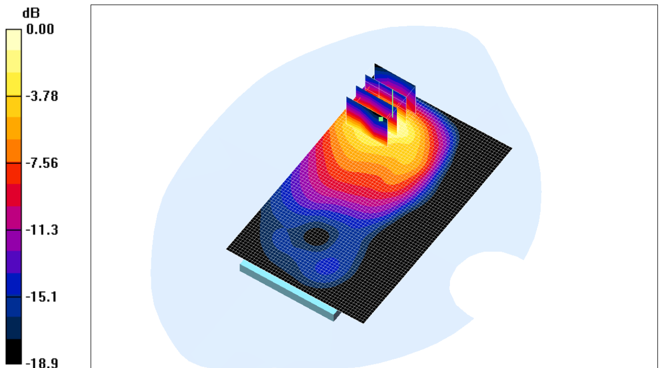
Fig. 11 : Distribution du DAS en WCDMA 2100: canal 9888 (1977.6 MHz) face arrière à 0.5cm du fantôme
