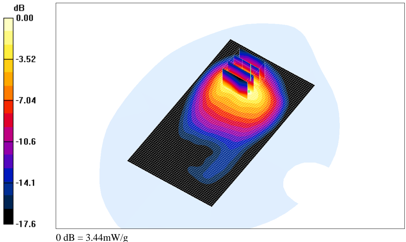
Fig. 13 : Distribution du DAS en LTE 1800: canal 19850 (1775.0 MHz) face arrière à 0.5cm du fantôme
