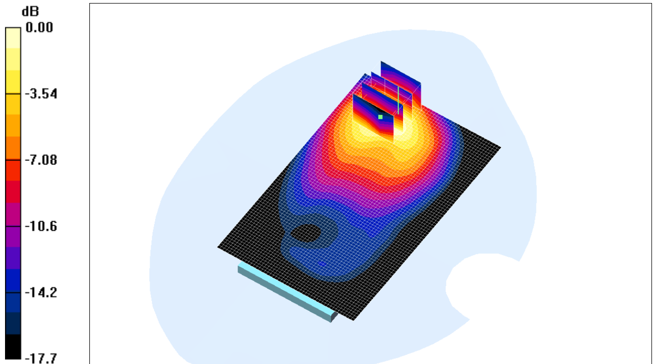
Fig. 9 : Distribution du DAS en GSM-GPRS 1800: canal 699 (1747.6 MHz) face arrière à 0.5cm du fantôme
