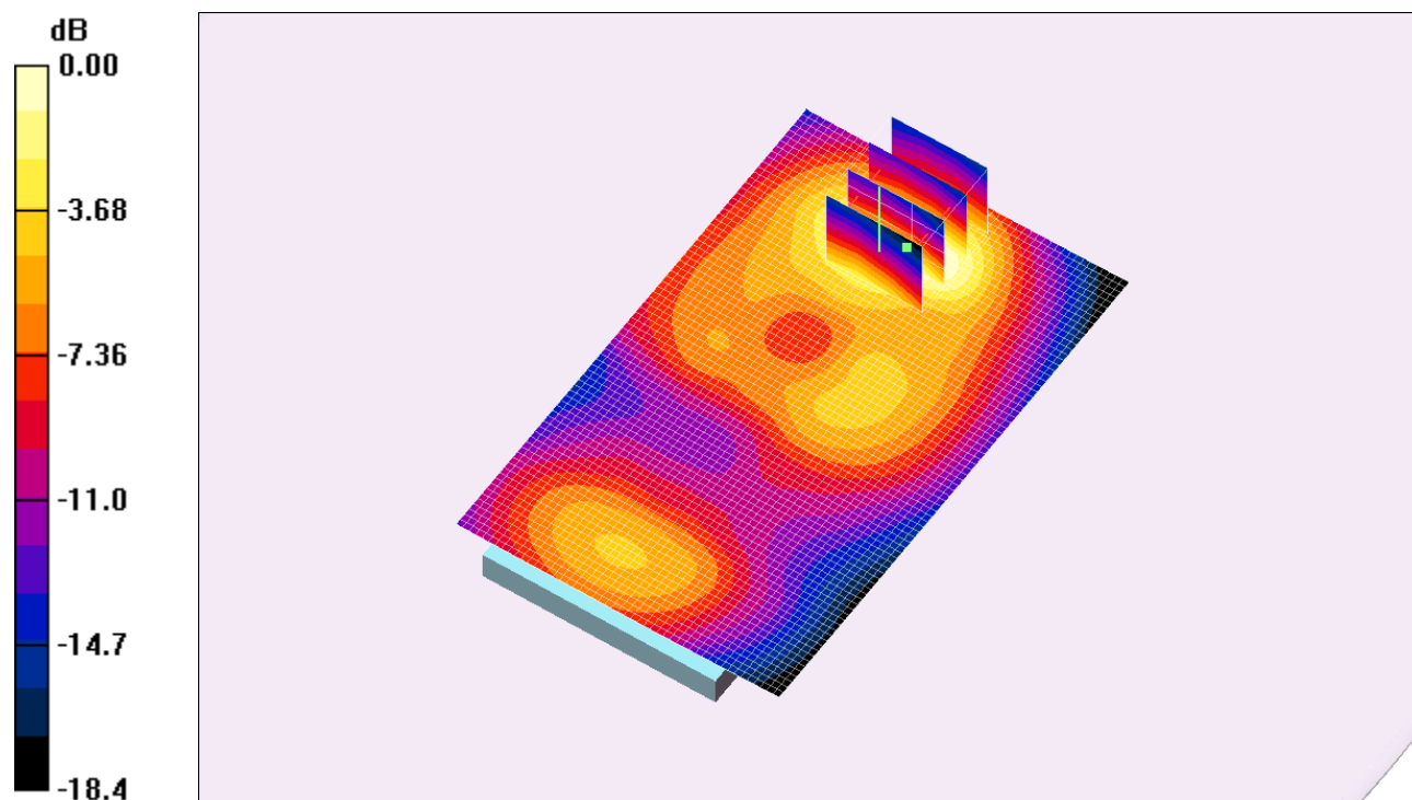
Fig. 11: Distribution du DAS en WCDMA 2100: canal 9888 (1977.6 MHz) face arrière à 1.5cm du fantôme
