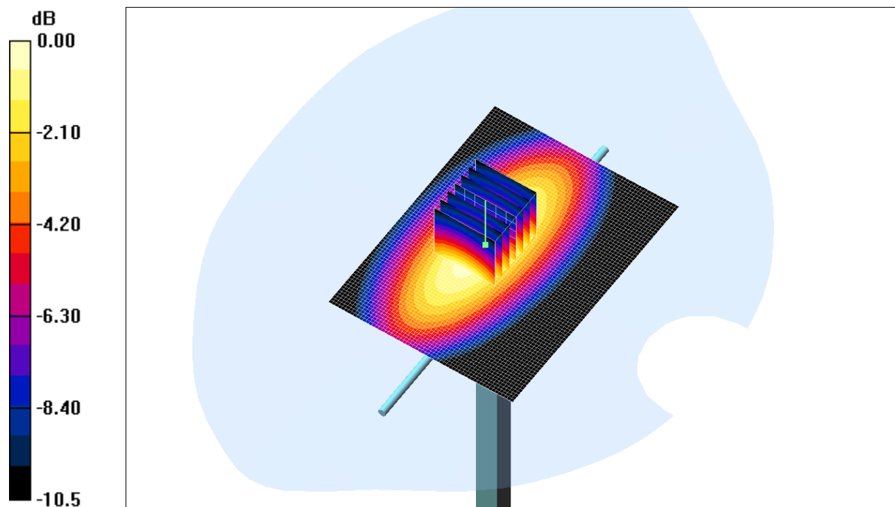
Fig. 3: Résultat de la vérification à 835MHz
