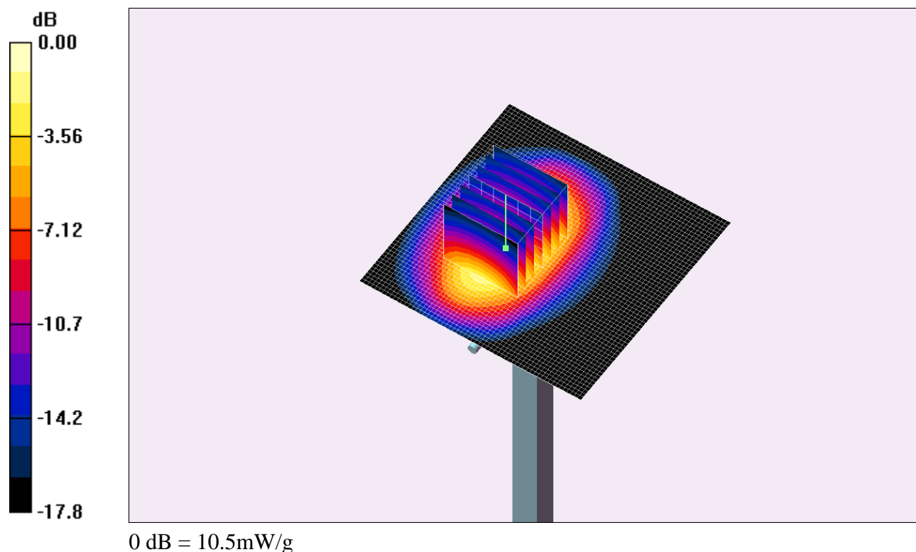
Fig. 5: Résultat de la vérification à 1800MHz
