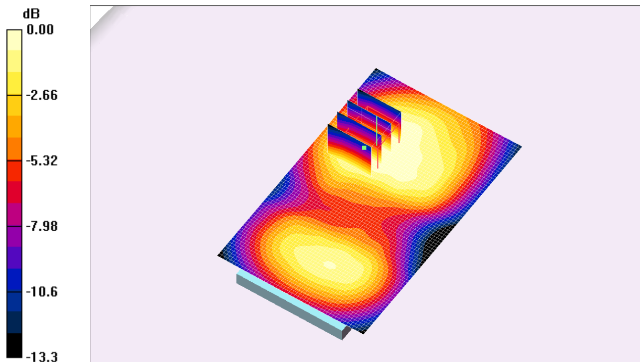
Fig. 9: Distribution du DAS en GSM-GPRS 1800: canal 699 (1747.6 MHz) face avant à 1.5cm du fantôme
