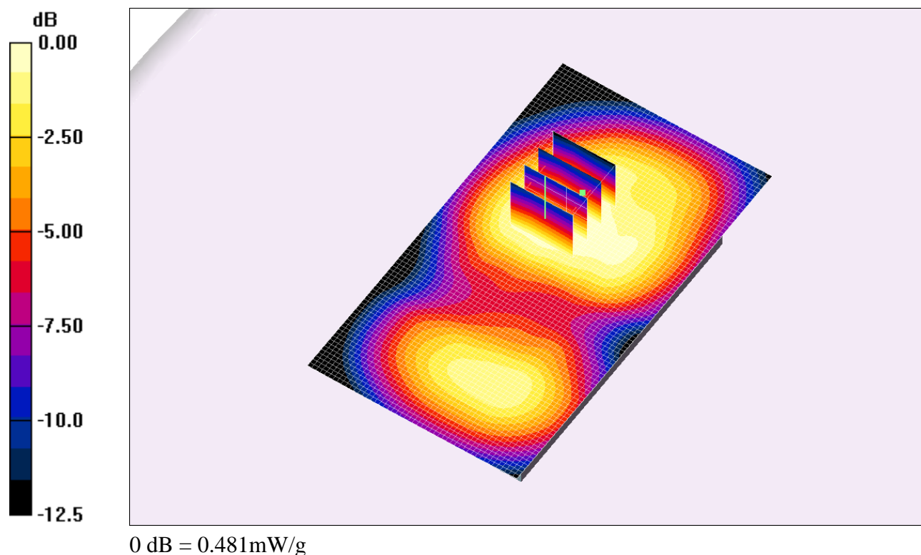
Fig. 13: Distribution du DAS en LTE 1800: canal 19575 (1747.5 MHz) face avant à 1.5cm du fantôme
