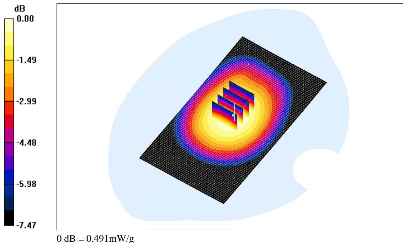
Fig. 12: Distribution du DAS en LTE 800: canal 24350 (852.0 MHz) face arrière à 1.5cm du fantôme
