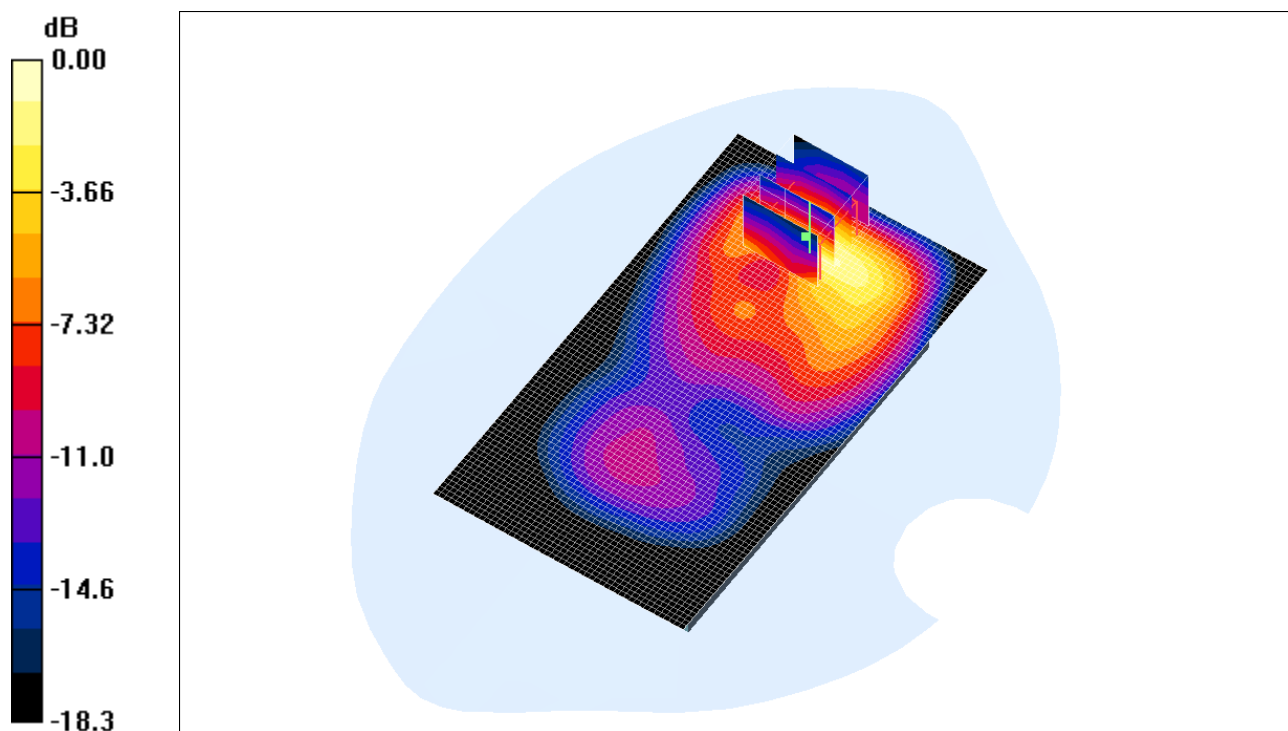
Fig. 13: Distribution du DAS en LTE 1800: canal 19300 (1720.0 MHz) face arrière à 0.5cm du fantôme
