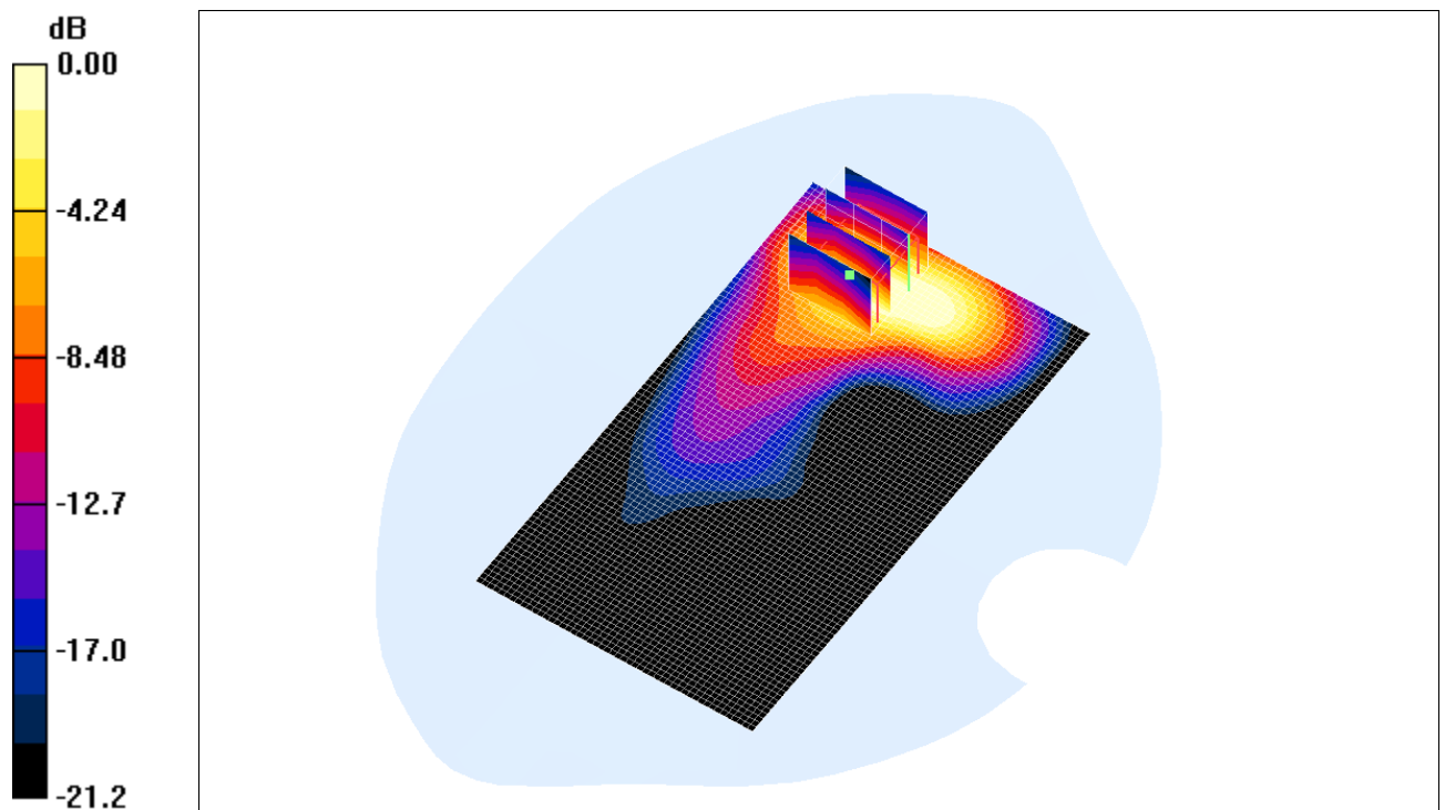
Fig. 14 : Distribution du DAS en LTE 2600: canal 20850 (2510.0 MHz) face arrière à 0.5cm du fantôme
