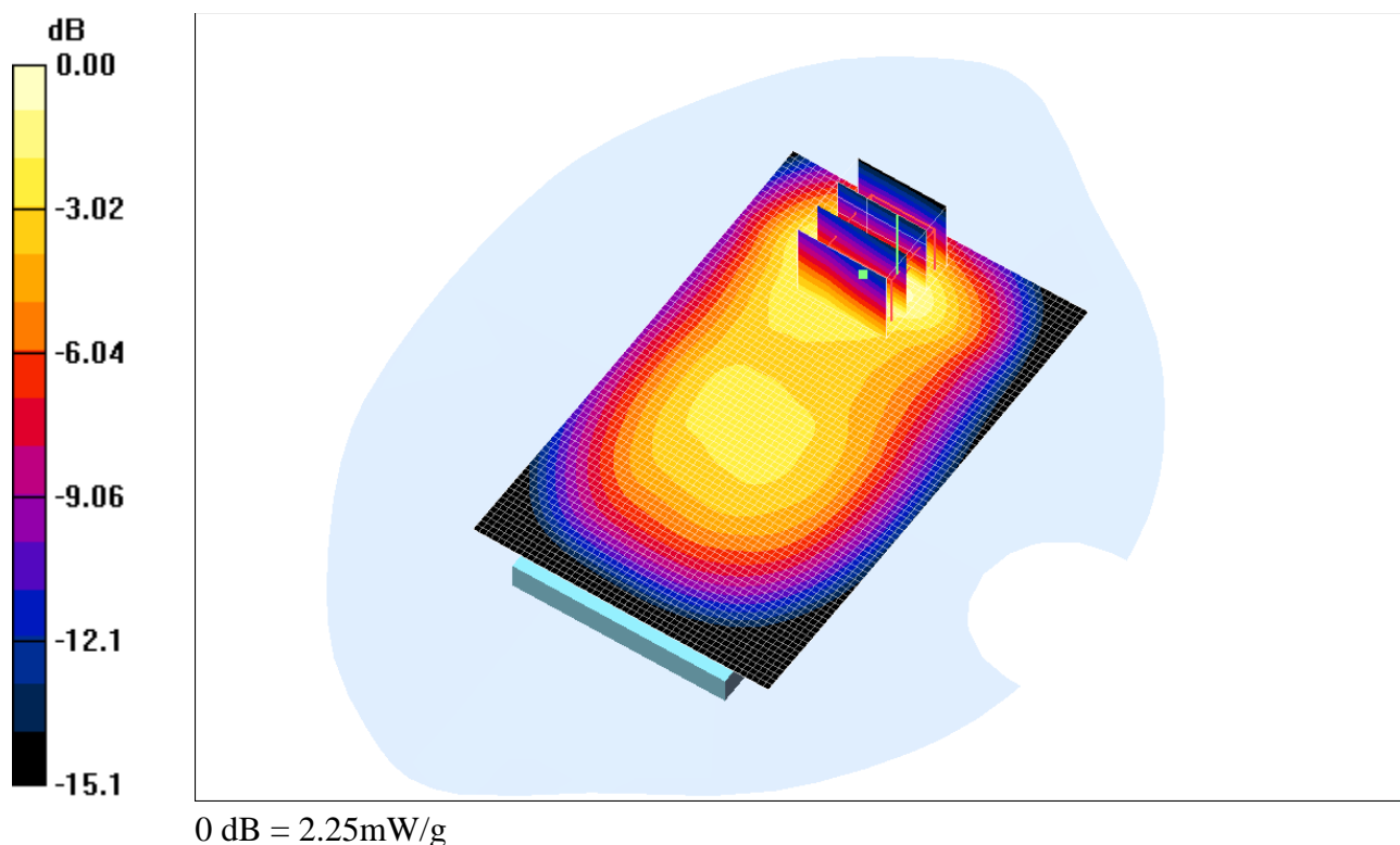
Fig. 8: Distribution du DAS en GSM-GPRS 900: canal 038 (897.6 MHz) face arrière à 0.5cm du fantôme
