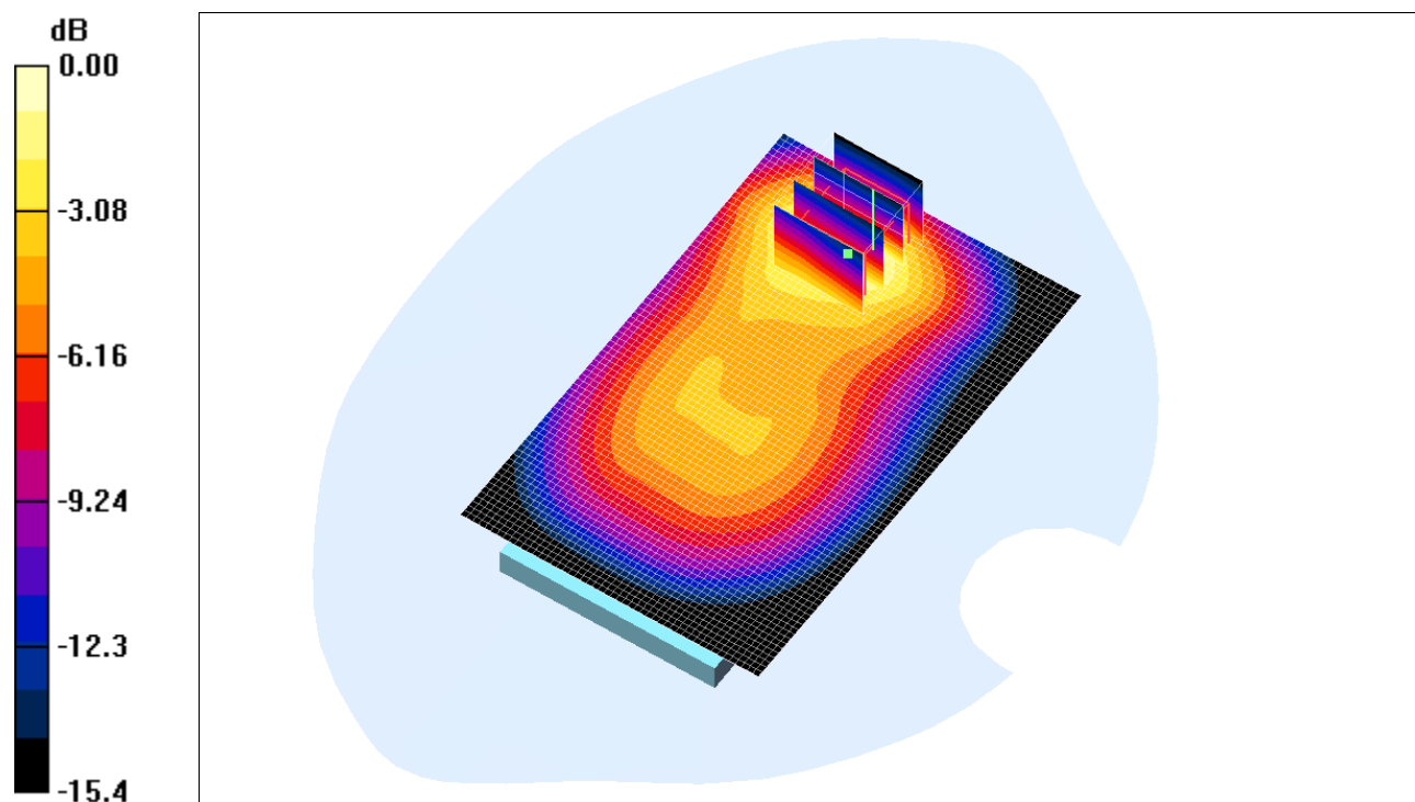
Fig. 10: Distribution du DAS en WCDMA 900: canal 2863 (912.6 MHz) face arrière à 0.5cm du fantôme
