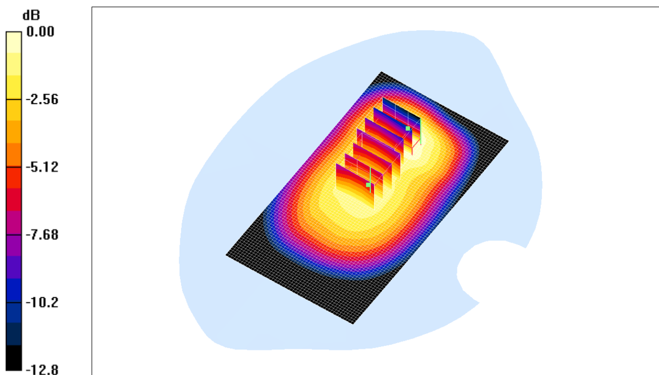
Fig. 12: Distribution du DAS en LTE 800: canal 24350 (852.0 MHz) face arrière à 0.5cm du fantôme
