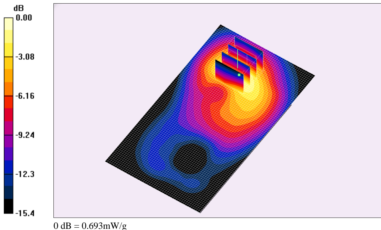
Fig. 13: Distribution du DAS en LTE 1800: canal 19850 (1775.0 MHz) face arrière à 1.5cm du fantôme
