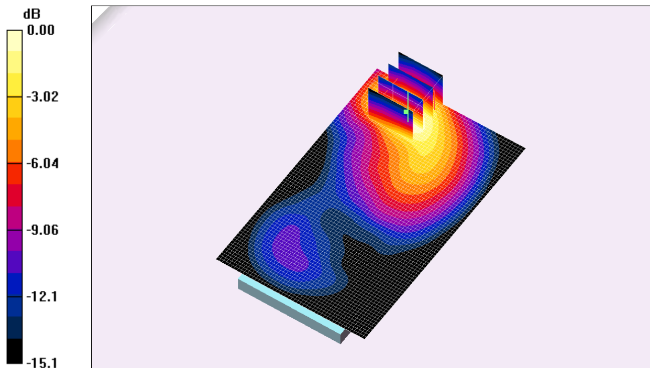
Fig. 9: Distribution du DAS en GSM-GPRS 1800: canal 699 (1747.6 MHz) face arrière à 1.5cm du fantôme
