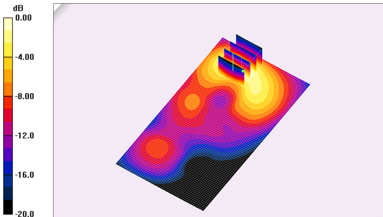
Fig. 14: Distribution du DAS en LTE 2600: canal 20850 (2510.0 MHz) face arrière à 1.5cm du fantôme
