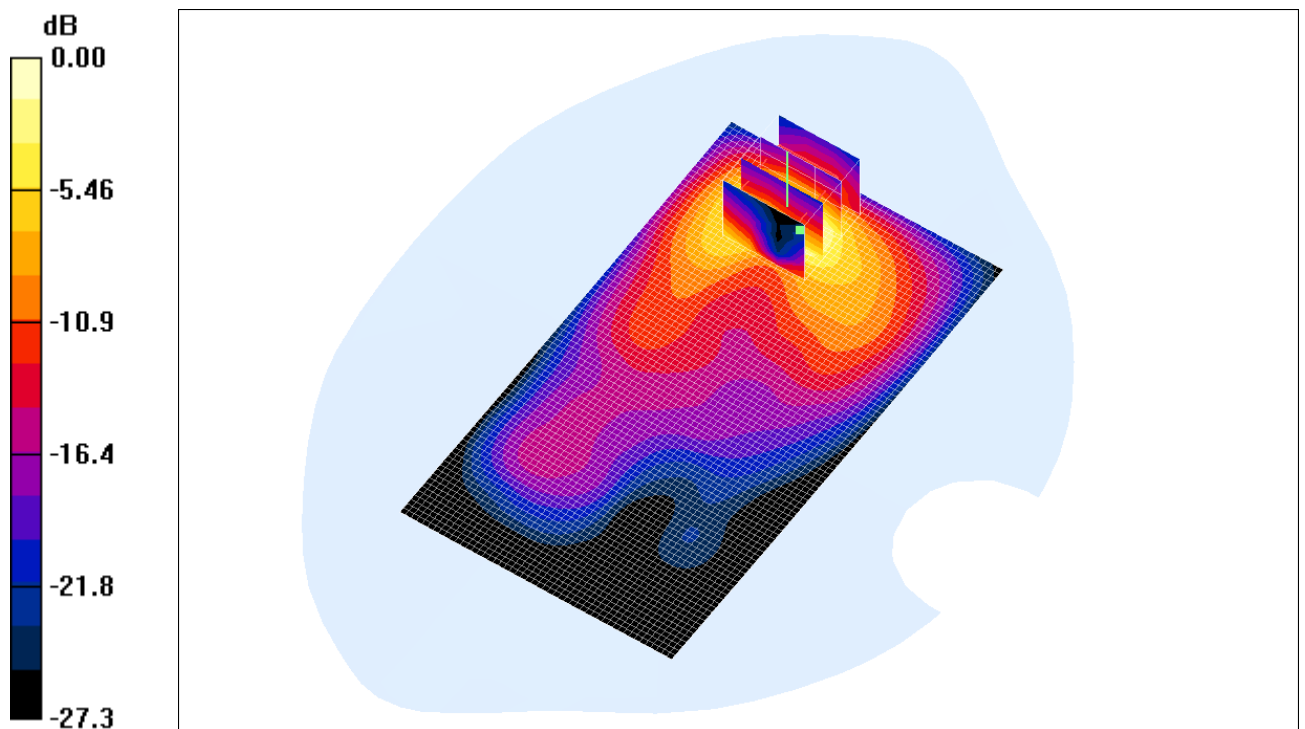
Fig. 14: Distribution du DAS en LTE 2600: canal 21100 (2535.0 MHz) face arrière à 0.5cm du fantôme
