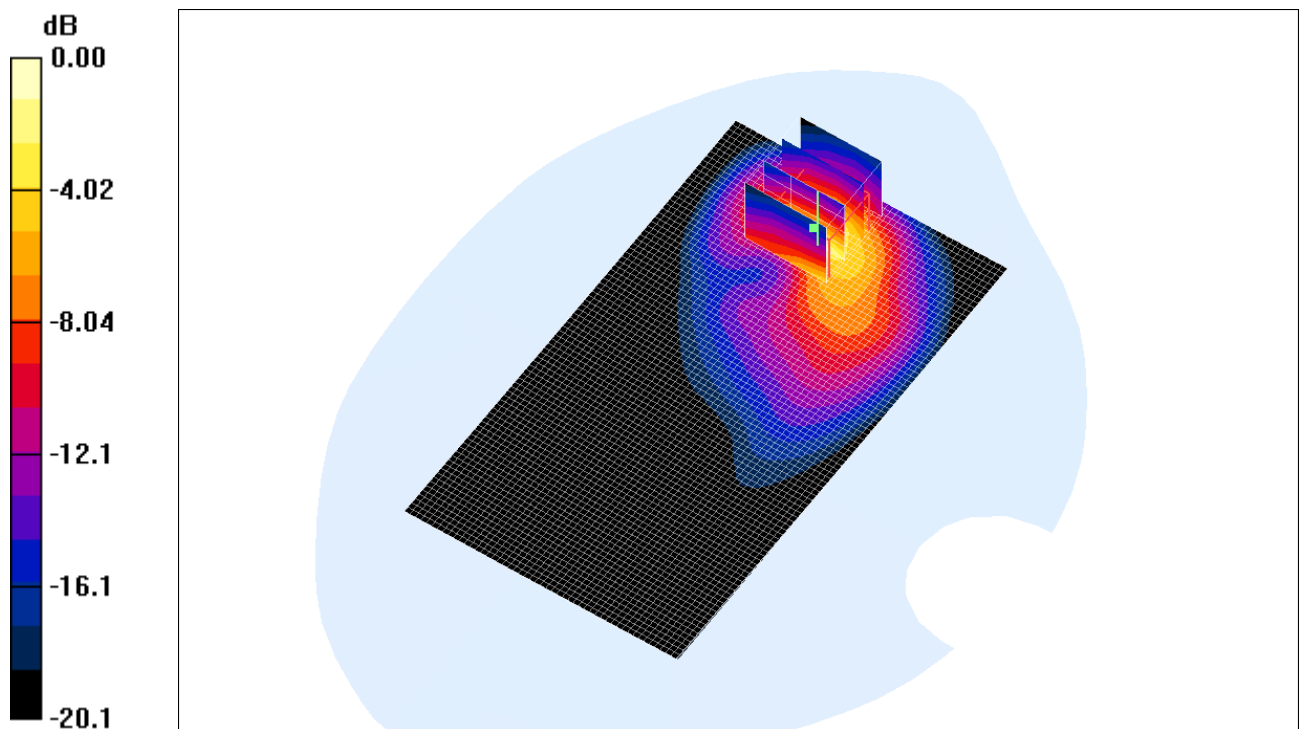
Fig. 13: Distribution du DAS en LTE 1800: canal 19575 (1747.5 MHz) face arrière à 0.5cm du fantôme
