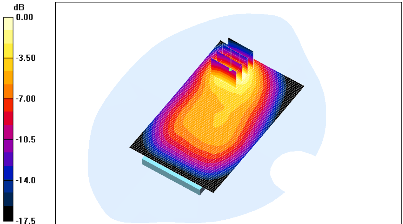
Fig. 10: Distribution du DAS en WCDMA 900: canal 2788 (897.6 MHz) face arrière à 0.5cm du fantôme
