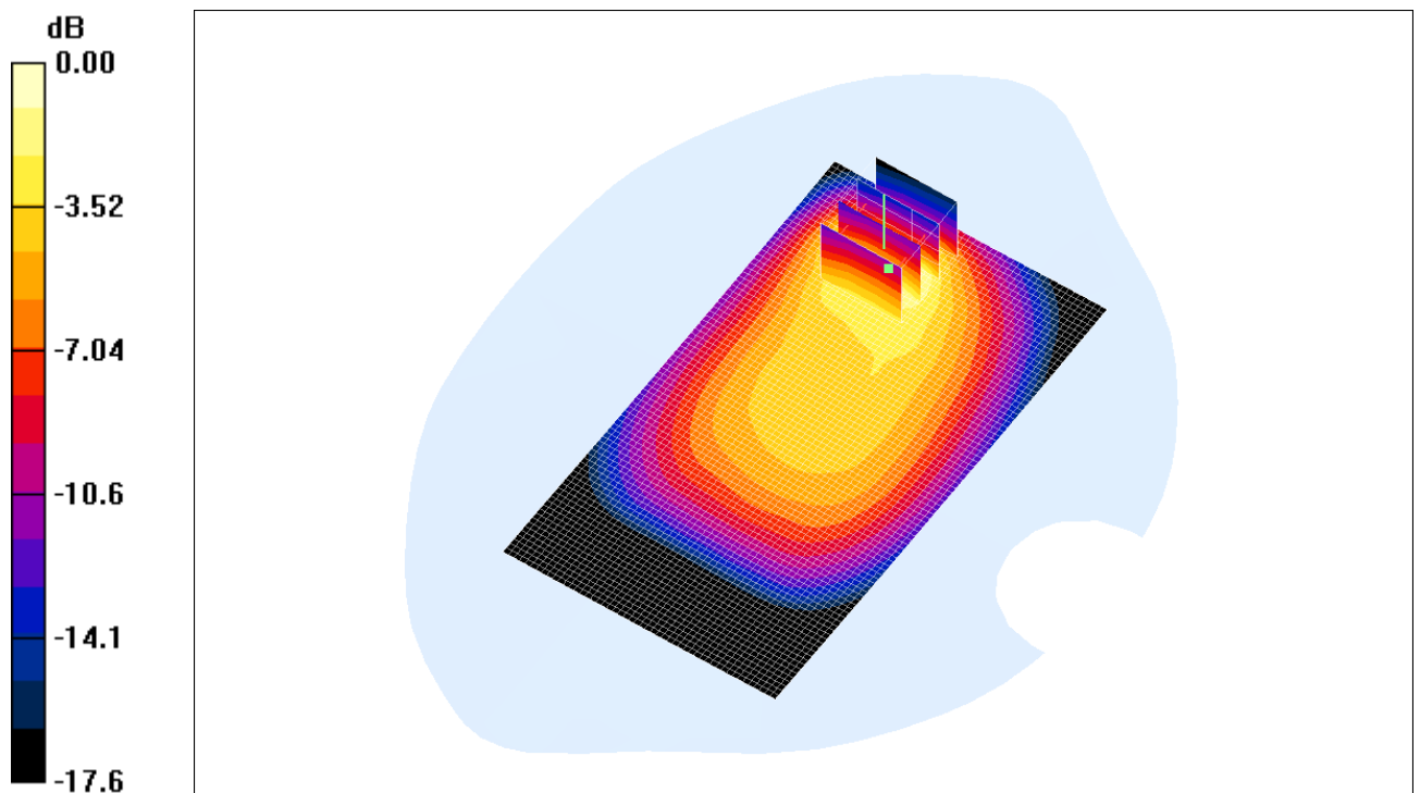
Fig. 12: Distribution du DAS en LTE 800: canal 24250 (842.0 MHz) face arrière à 0.5cm du fantôme
