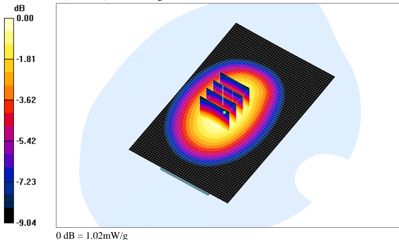
Fig. 5: Distribution du DAS en GSM 900: canal 124 (914.8 MHz) face arrière à 1.5cm du fantôme
