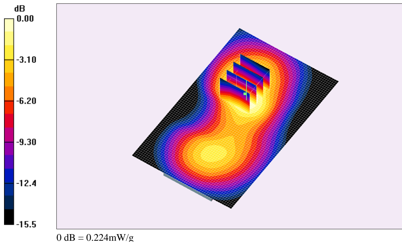
Fig. 6: Distribution du DAS en GSM 1800: canal 885 (1784.8 MHz) face avant à 1.5cm du fantôme
