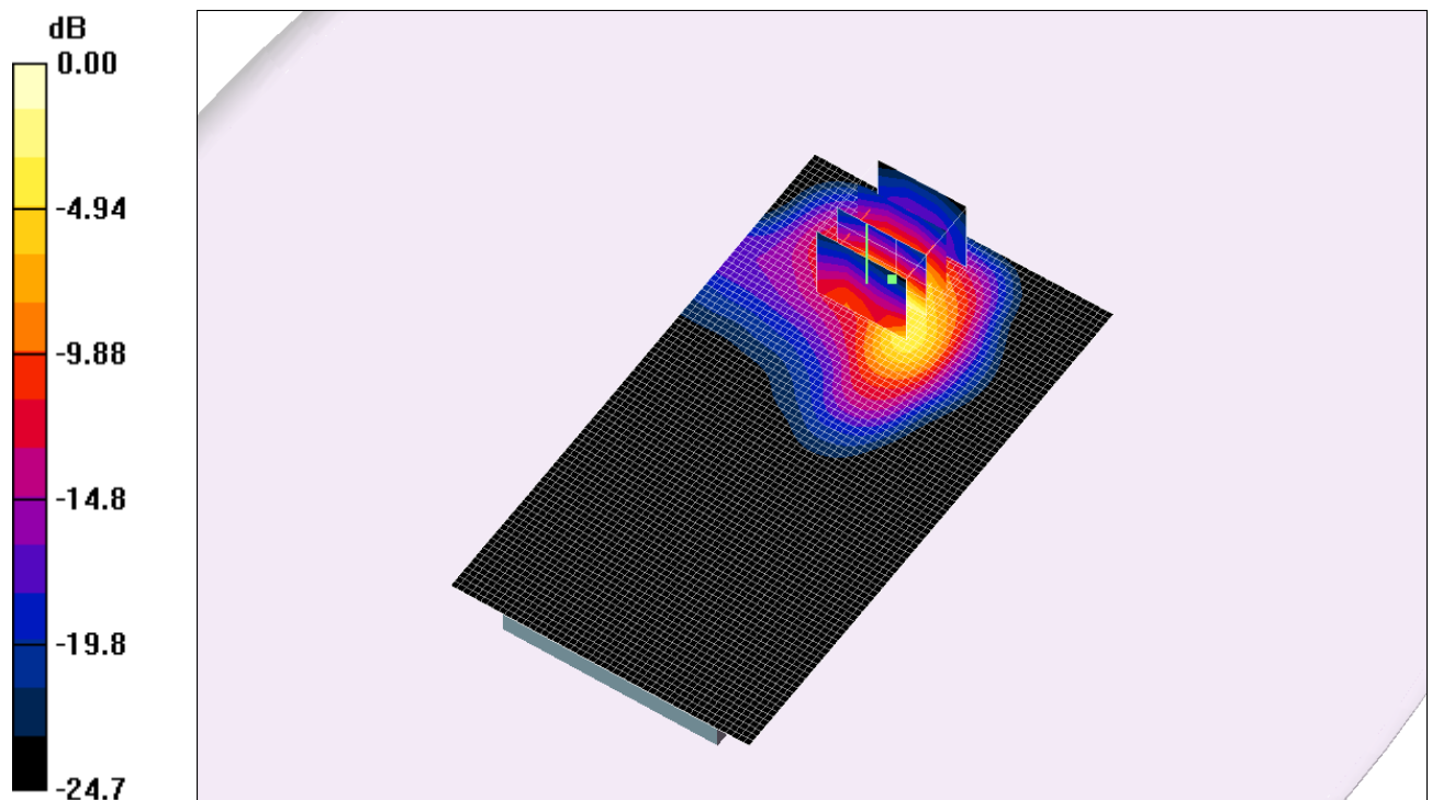
Fig. 14: Distribution du DAS en LTE 2600: canal 20850 (2510.0 MHz) face avant à 0cm du fantôme
