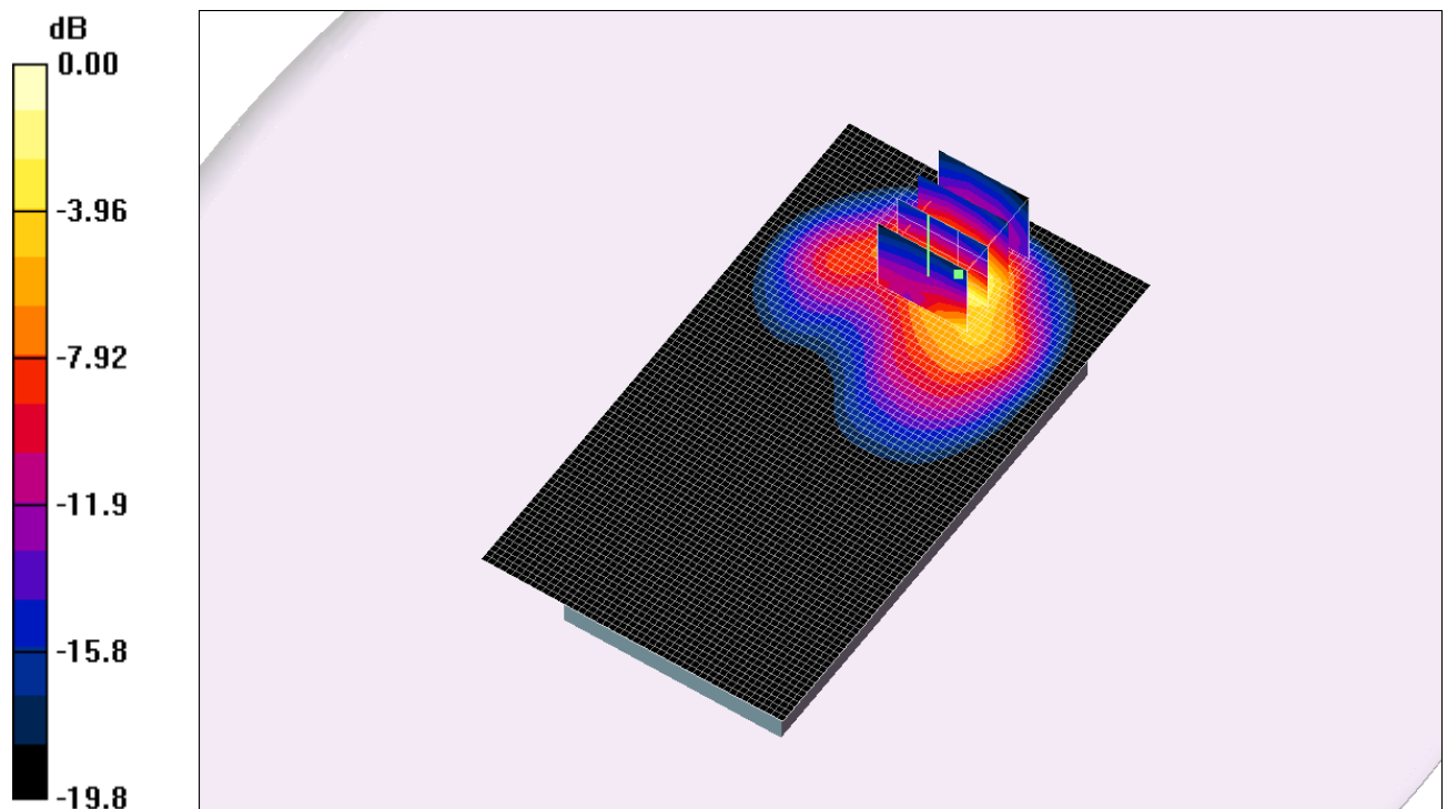
Fig. 13: Distribution du DAS en LTE 1800: canal 19925 (1782.5 MHz) face avant à 0cm du fantôme
