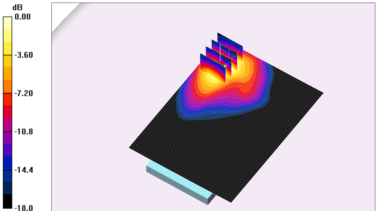
Fig. 9: Distribution du DAS en GSM-GPRS 1800: canal 699 (1747.6 MHz) face arrière à 0cm du fantôme
