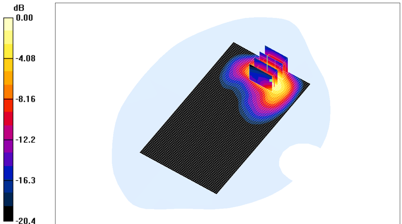
Fig. 11: Distribution du DAS en WCDMA 2100: canal 9612 (1922.4 MHz) face avant à 0cm du fantôme
