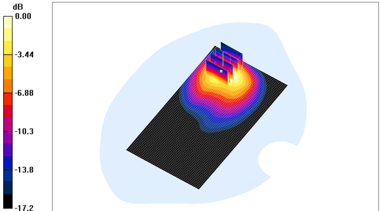
Fig. 12: Distribution du DAS en LTE 800: canal 24300 (847.0 MHz) face arrière à 0cm du fantôme
