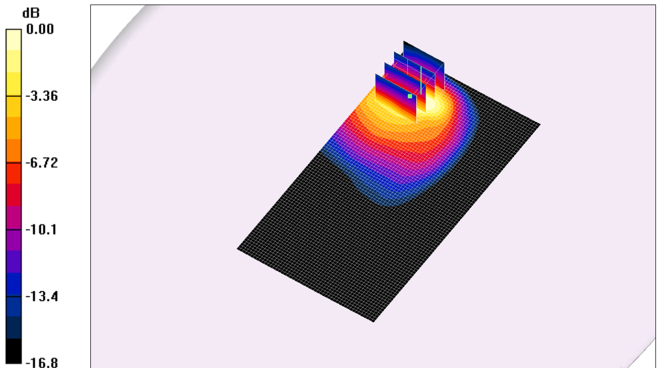
Fig. 10: Distribution du DAS en WCDMA 900: canal 2863 (912.6 MHz) face arrière à 0cm du fantôme
